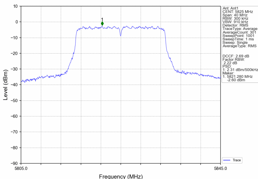
802.11n(HT20)_HCH_5825MHz_Ant1_NTNV
