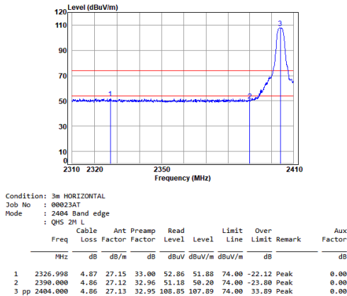
QHS_2M_TX_CH_01_Horizontal
