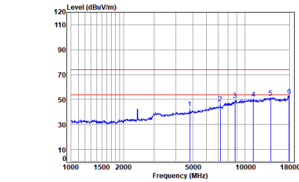
QHS_2M_TX_CH_01_Horizontal
