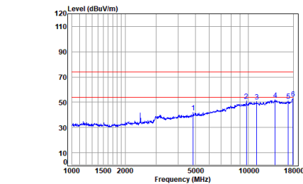
QHS_2M_TX_CH_19_Horizontal
