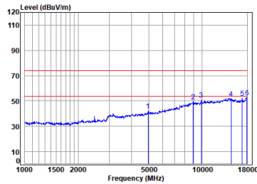
QHS_6M_TX_CH_01_Horizontal
