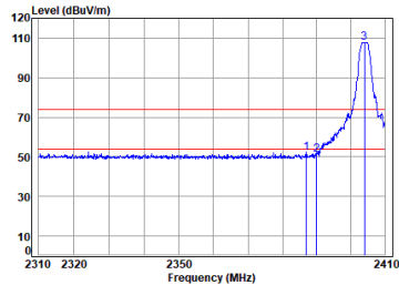
QHS_6M_TX_CH_01_Horizontal
