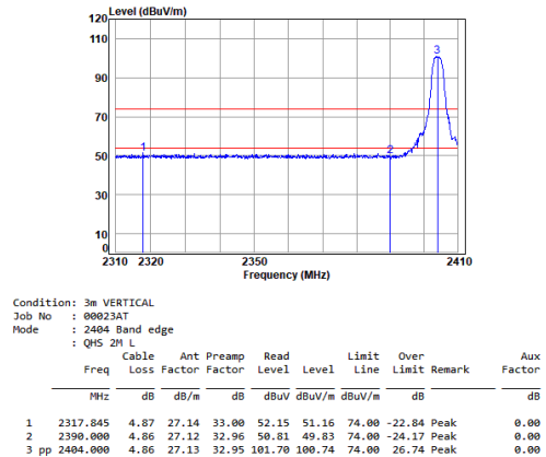
QHS_2M_TX_CH_01_Vertical
