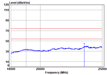
QHS_2M_TX_CH_38_Vertical
