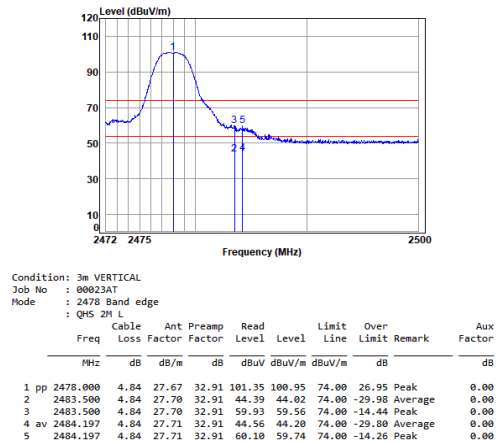
QHS_2M_TX_CH_38_Vertical
