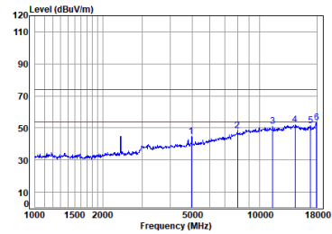
QHS_2M_TX_CH_01_Vertical
