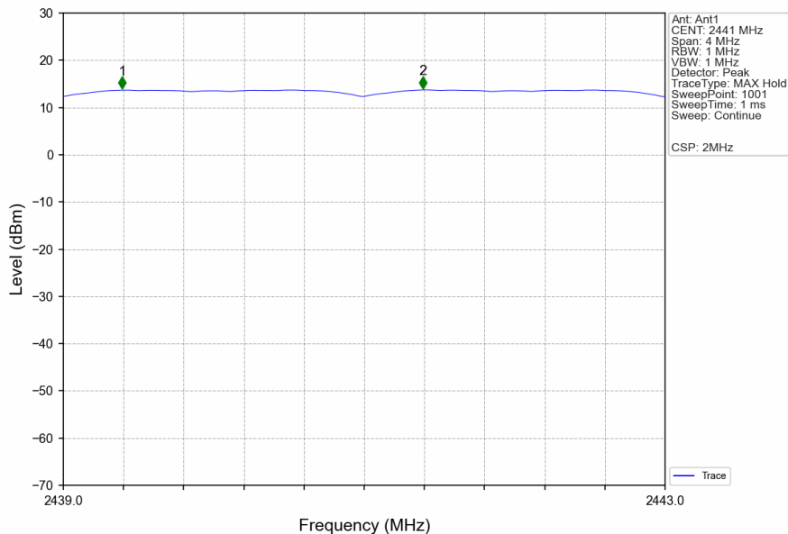
QHS 6M_HOPP_Ant1_NTNV
