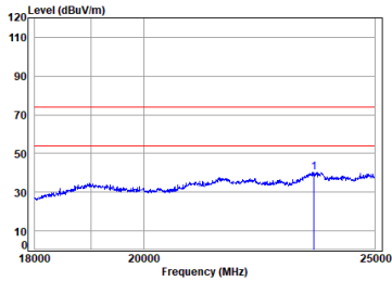
QHS_2M_TX_CH_38_Horizontal
