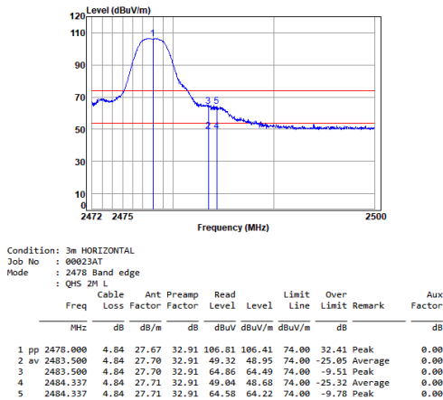
QHS_2M_TX_CH_38_Horizontal
