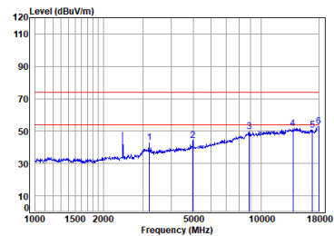
QHS_2M_TX_CH_19_Vertical
