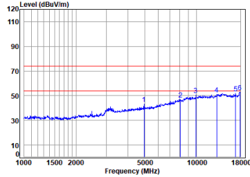
QHS_2M_TX_CH_38_Horizontal
