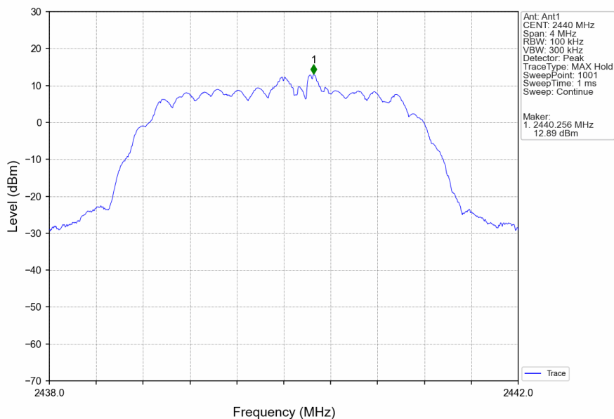
QHS 5M_MCH_2440MHz_Ant1_NTNV
