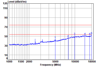
QHS_2M_TX_CH_38_Vertical
