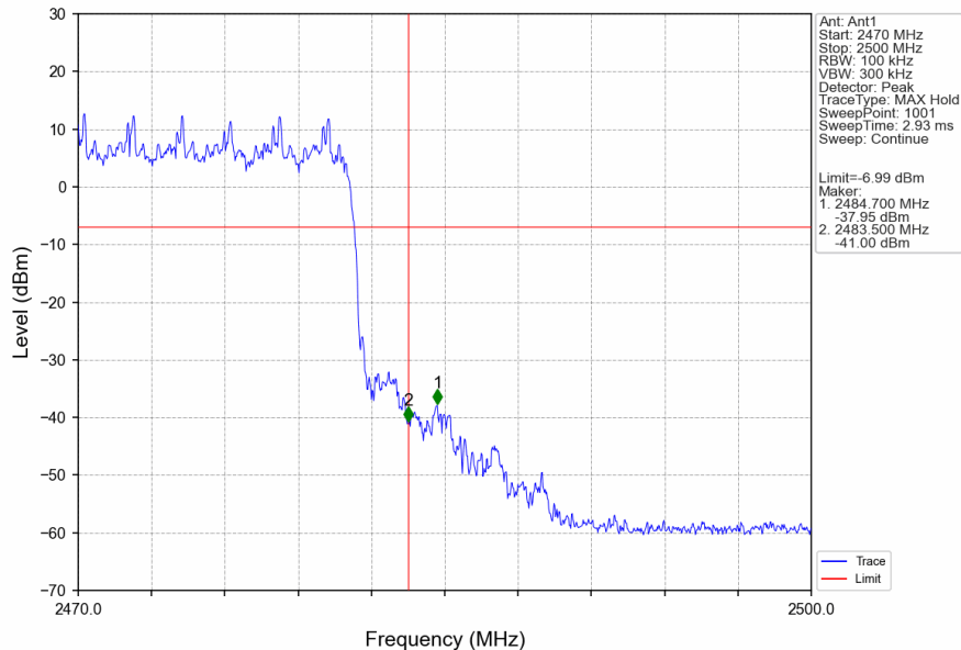
QHS 4M_HOPP_Ant1_NTNV
