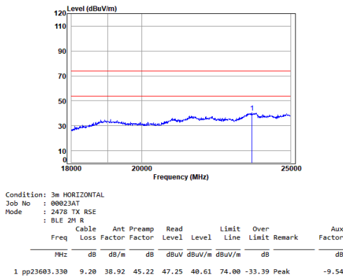
BLE_2M_TX_CH_38_Horizontal
