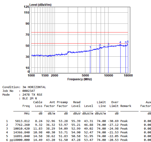
BLE_2M_TX_CH_38_Horizontal
