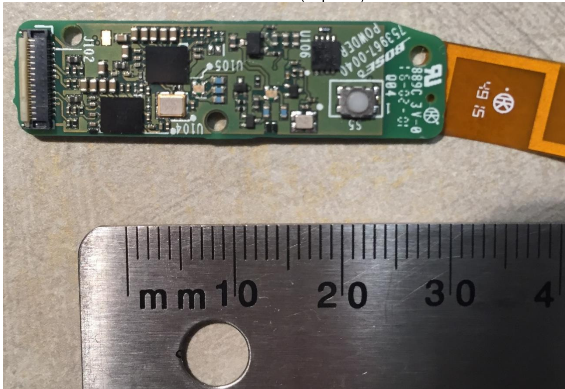
Bottom side
