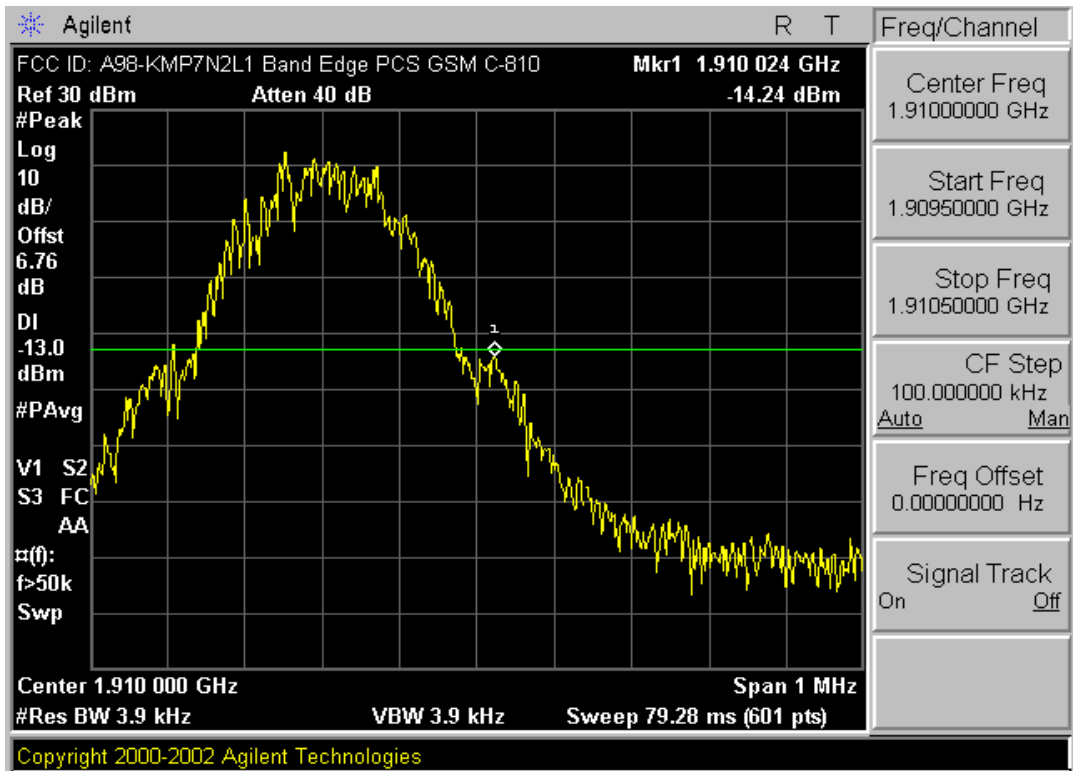
Plot A-9. Band Edge (PCS GSM – Ch. 810)
