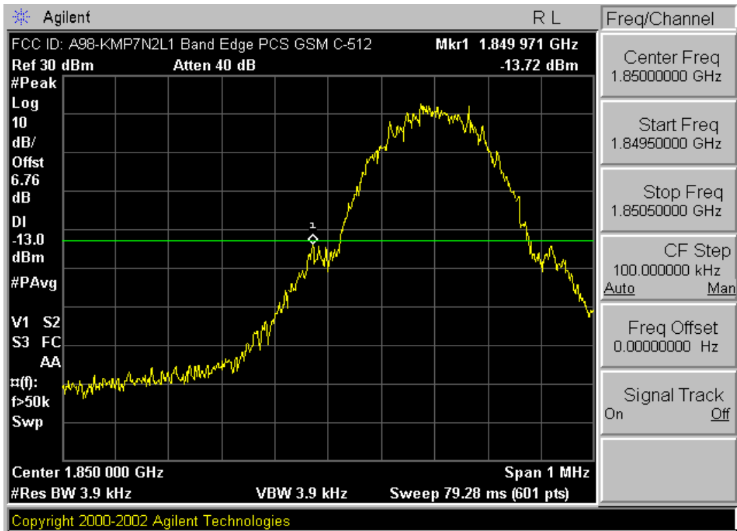
Plot A-3. Band Edge (PCS GSM – Ch. 512)
