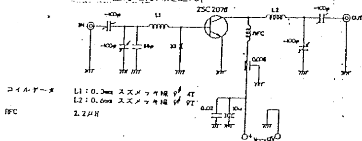
2SC2078 27MHz 出力電力測定回路
