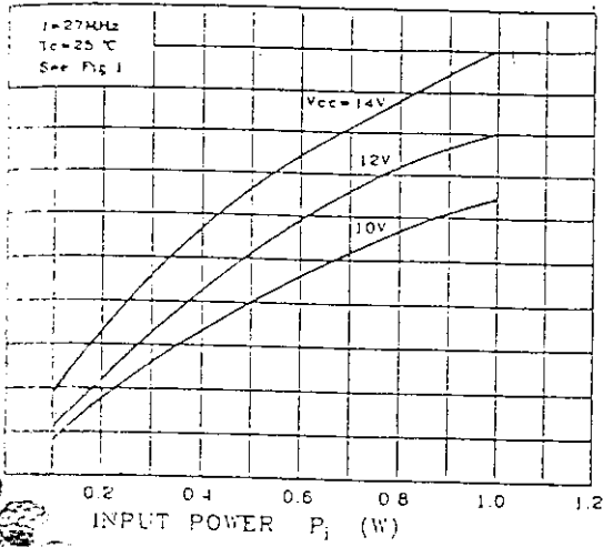
P_o - P_i
