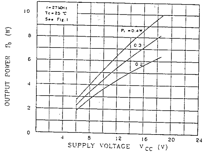
P_o - V_{cc}
