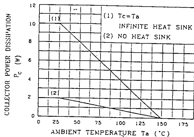
P_c - T_a
