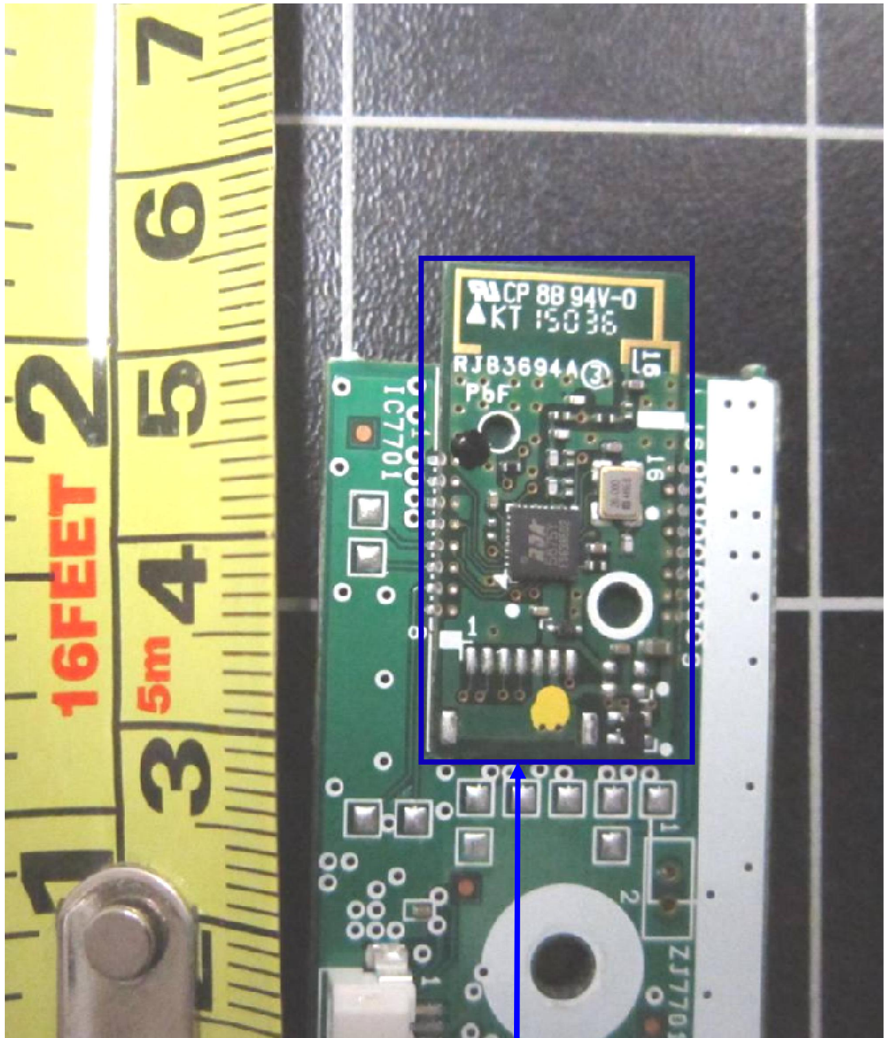
RF Module Circuit
