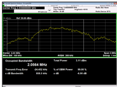
6dB 2440MHz
