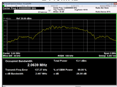
2440MHz
