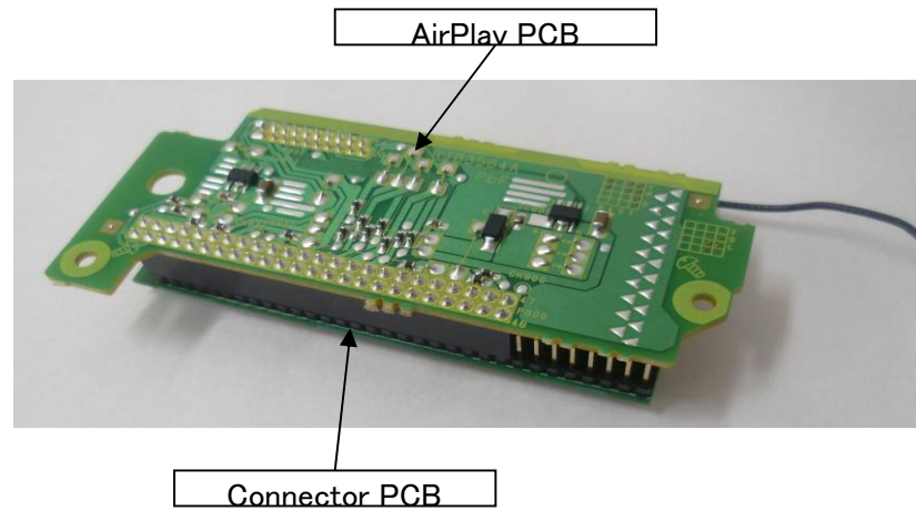
Wi-Fi Module
