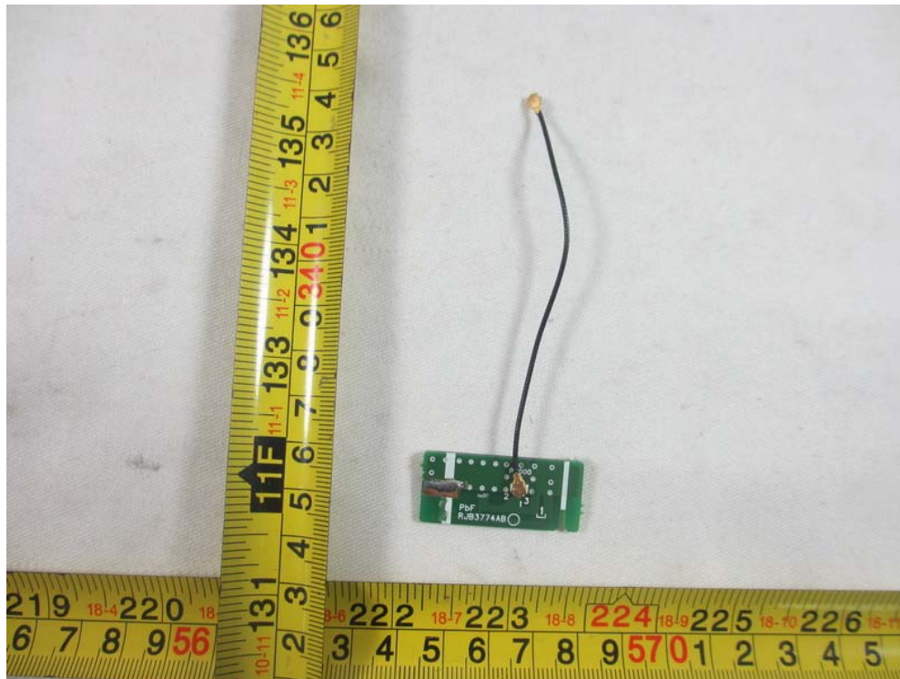
RF Module Ant 1
