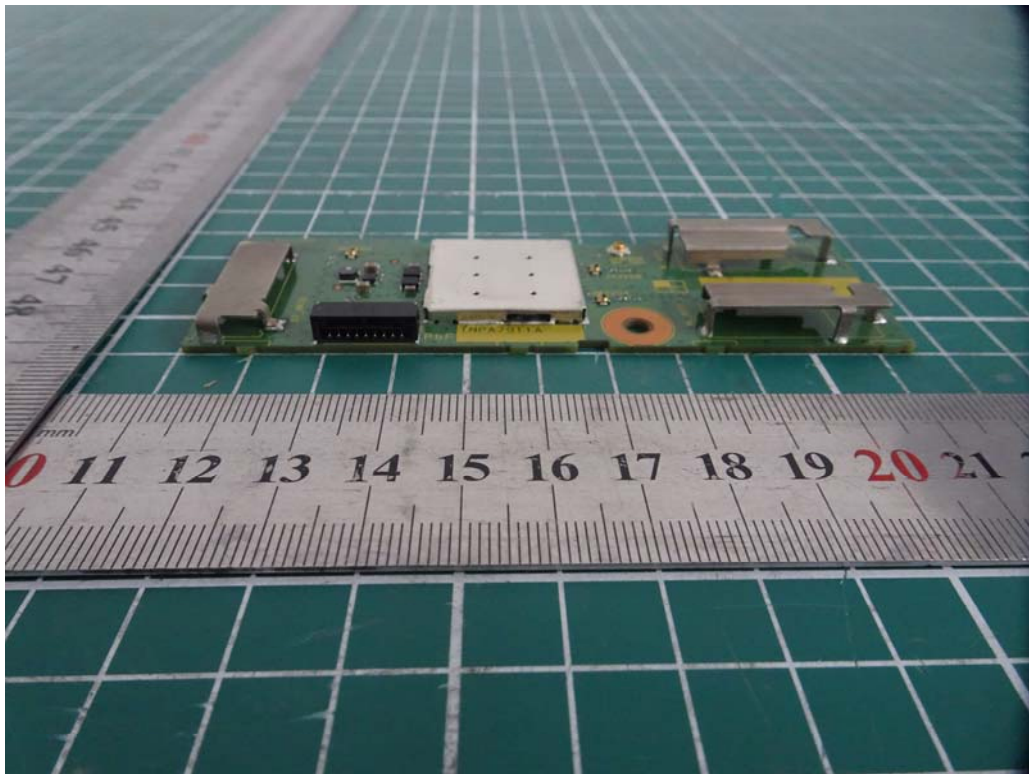
a: EUT
