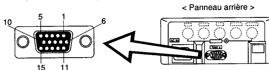
Affectation des broches de la miniprises à 15 broches D-Sub
