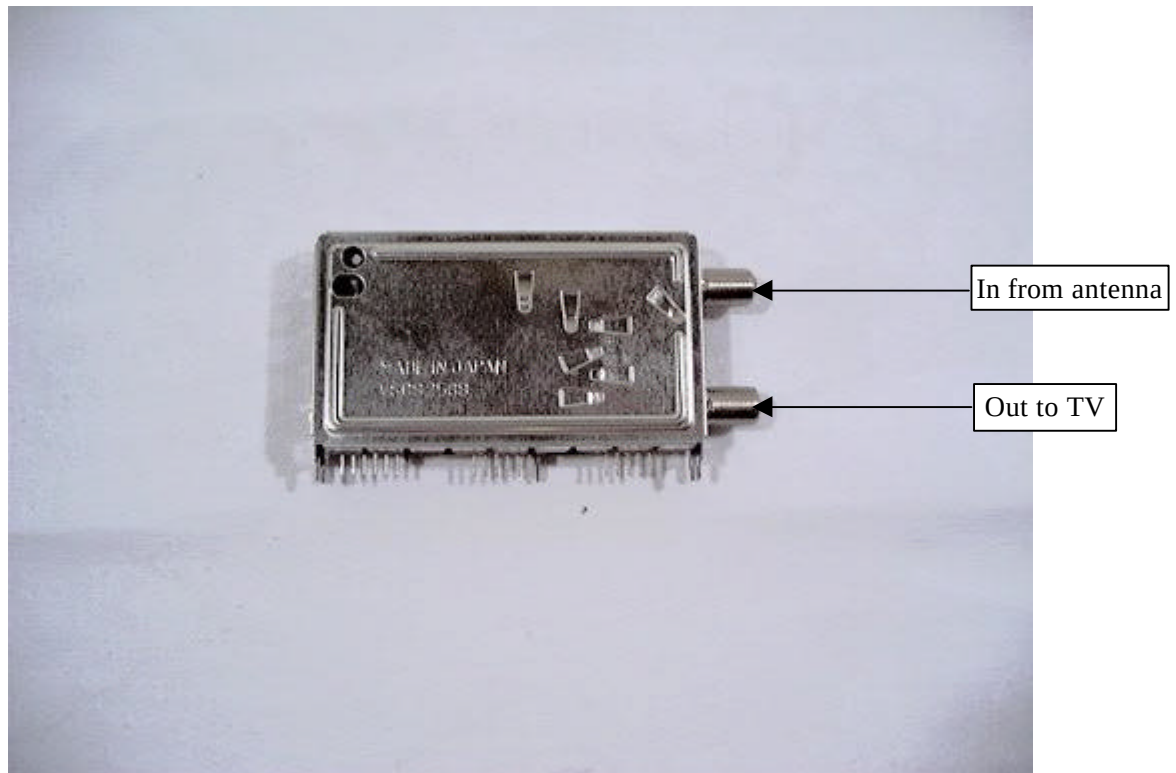
Tuner (VEQS0614: Top view)
