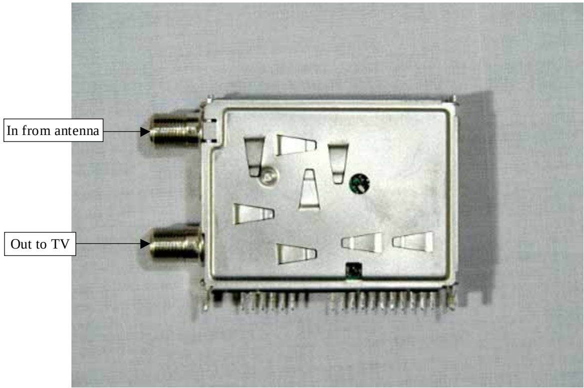
Tuner (ENG56D01G1: Top view)
