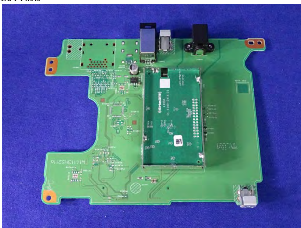
(47) EUT Photo
