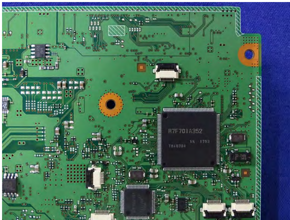
(74) EUT Photo
