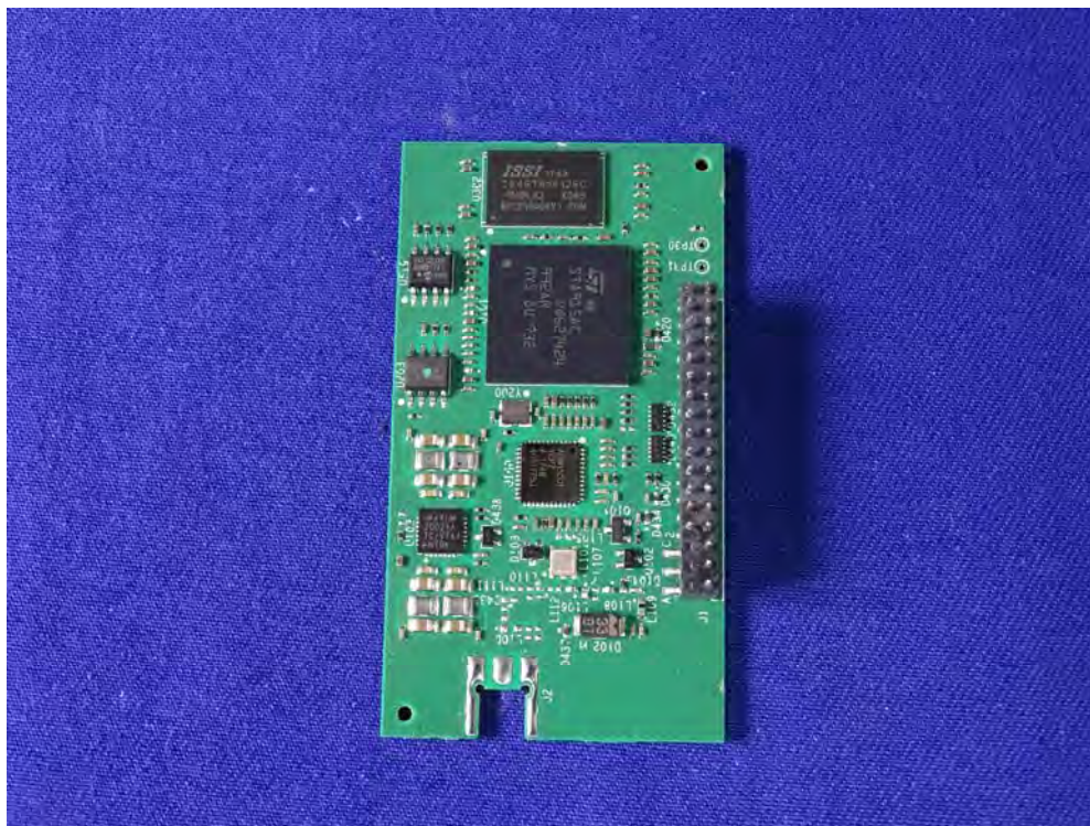
(52) EUT Photo
