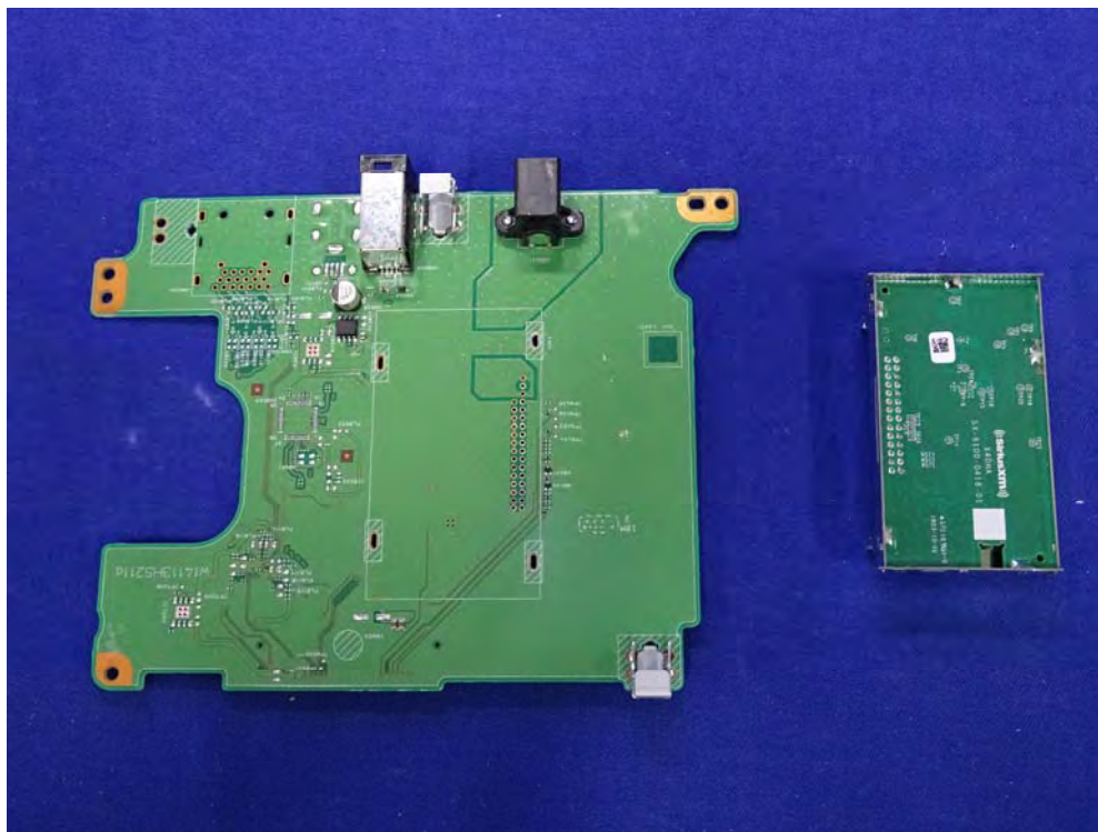
(48) EUT Photo
