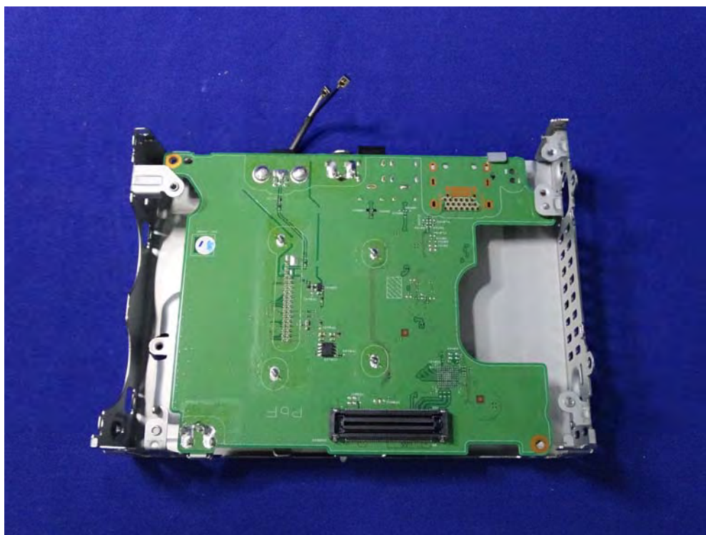
(41) EUT Photo
