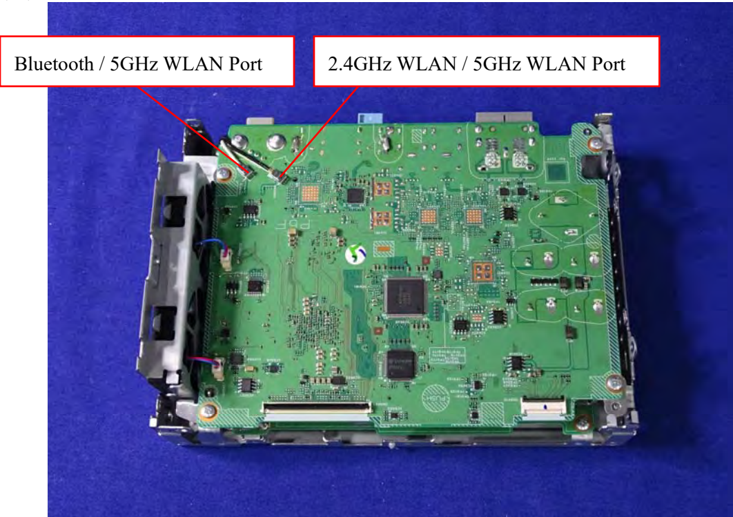
(15) EUT Photo
