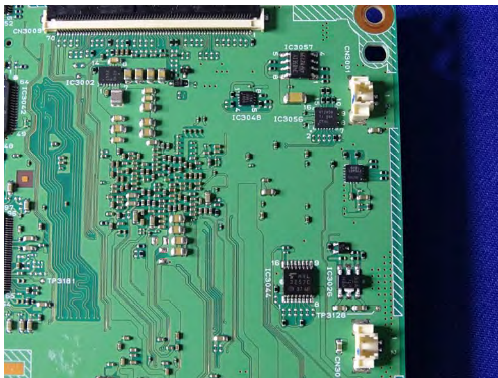
(36) EUT Photo
