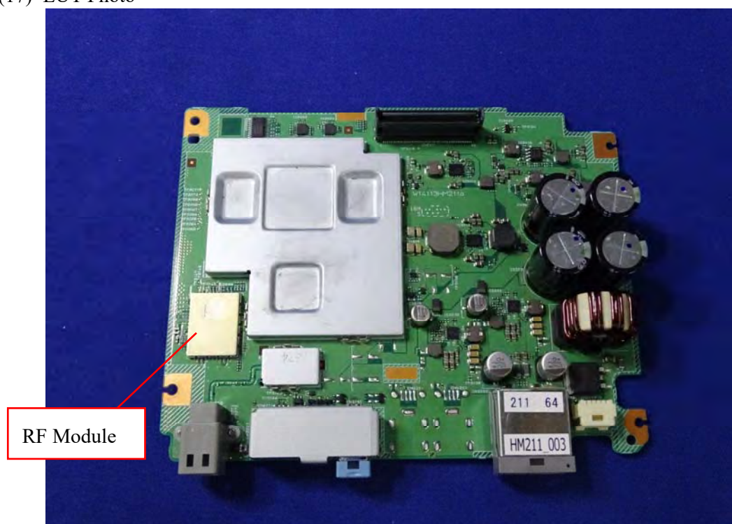
(17) EUT Photo
