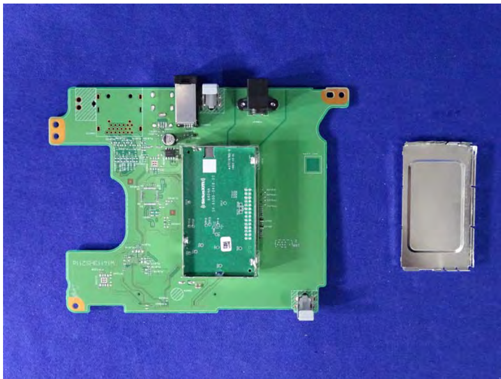
(46) EUT Photo
