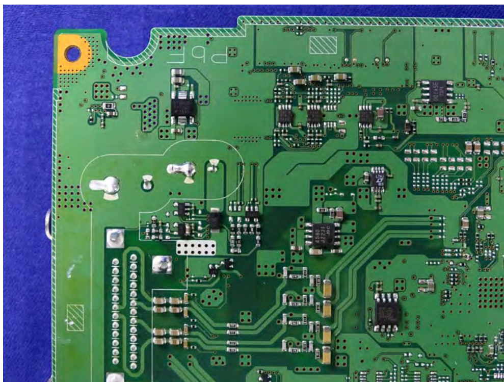
(71) EUT Photo
