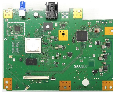
【SOC PCB / Solder Side】
