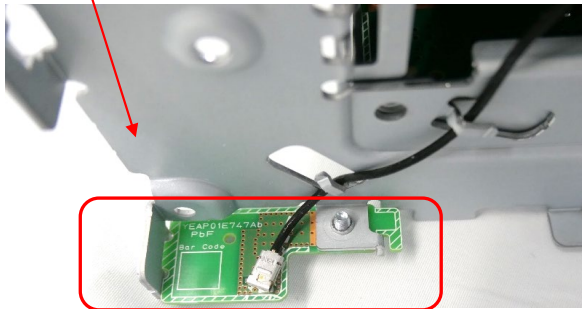
BT/wifi Antenna
