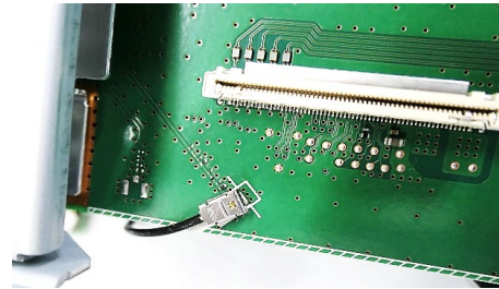
SOC PCB BT/wifi Antenna Input
