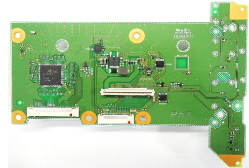
【TFT PCB / Solder Side】
