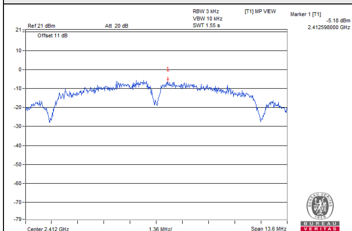
802.11b : CH 1
