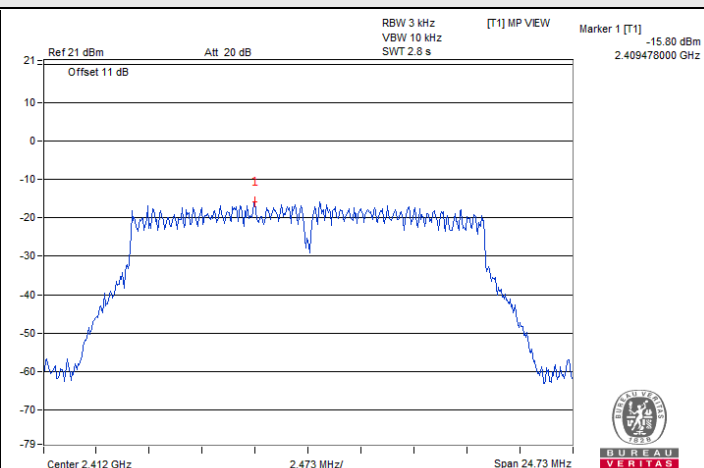
802.11g : CH 1
