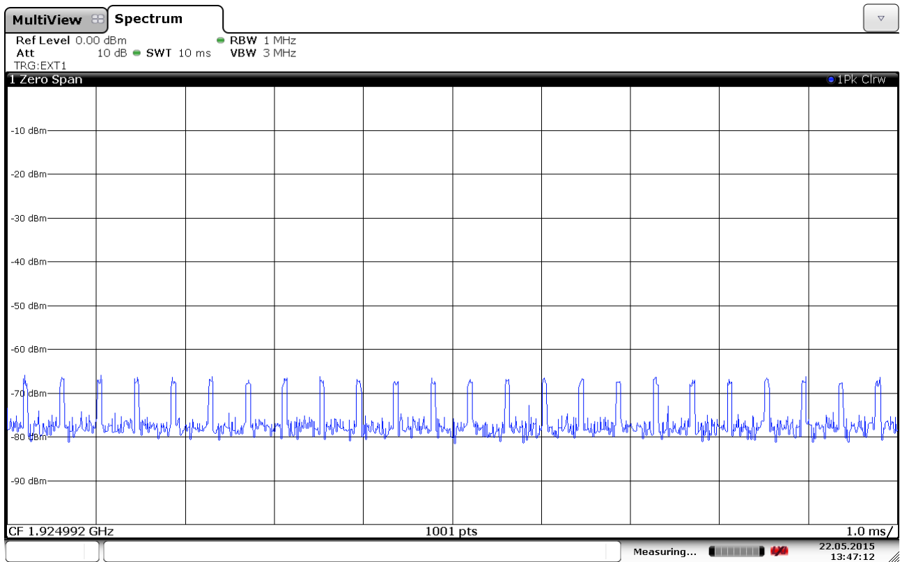
50 µs Pulses
