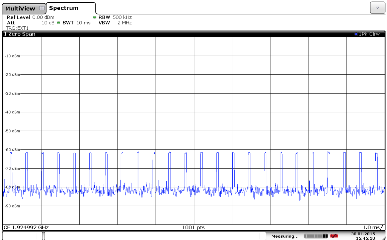
50 µs Pulses
