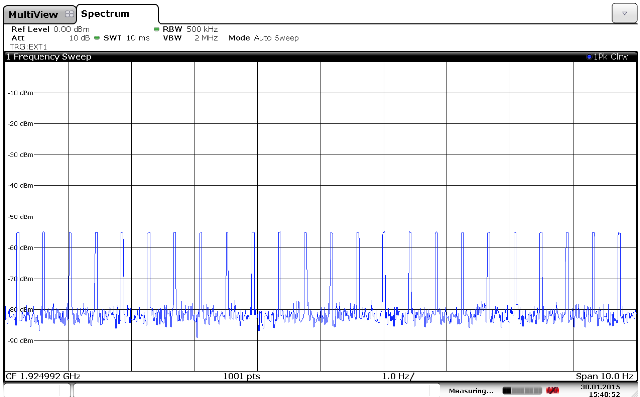
35 µs Pulses
