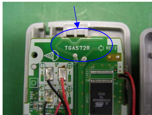
Antenna
