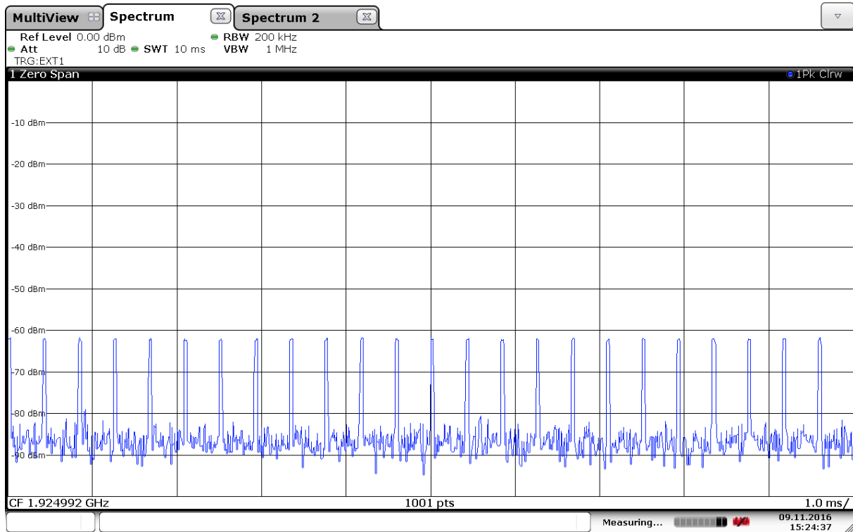
35 µs Pulses
