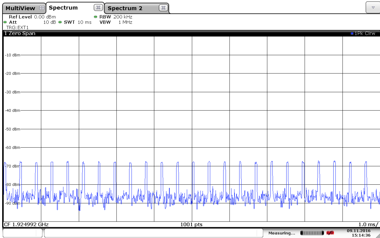
50 µs Pulses
