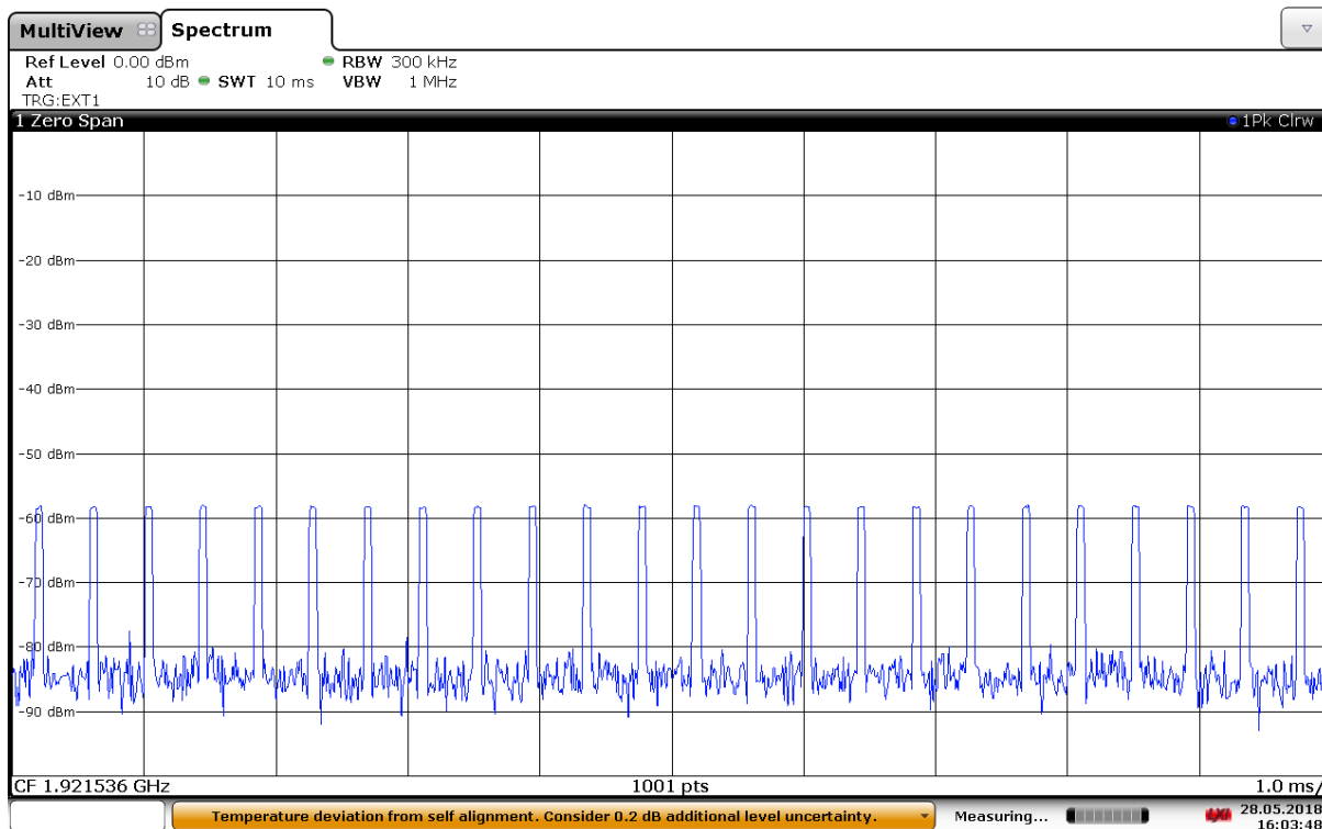
50 µs Pulses
