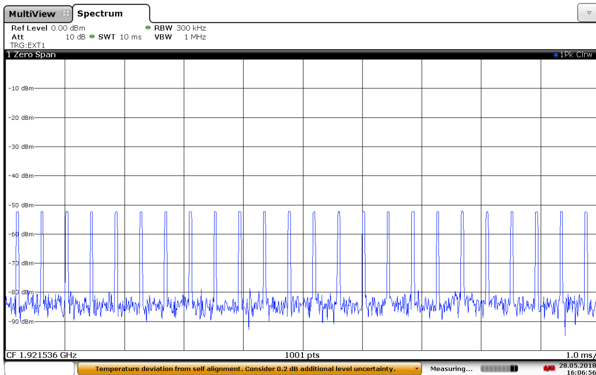
35 µs Pulses
