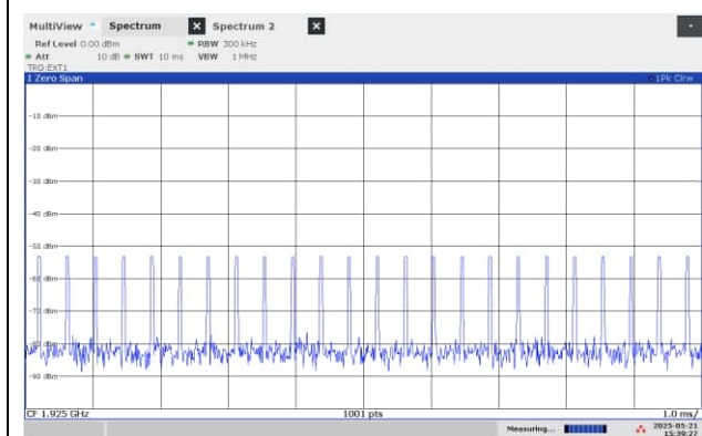
35 µs Pulses
