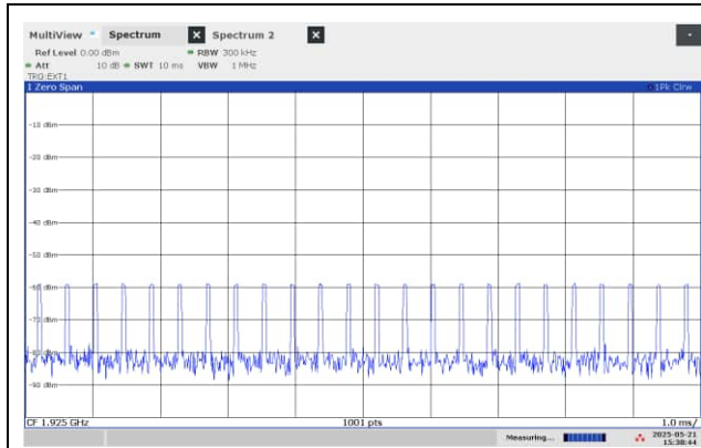
50 µs Pulses
