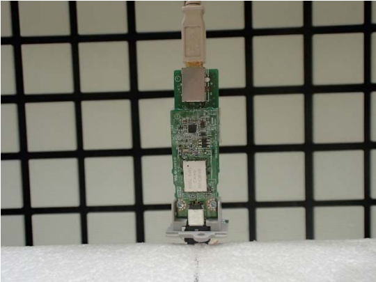
Module Z-axis
