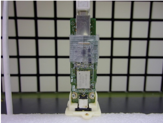
Module Z-axis
