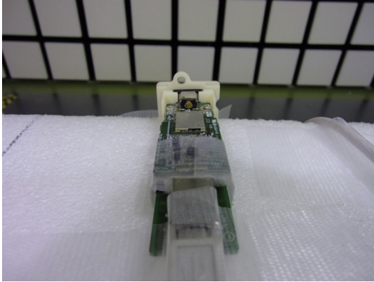
Module Y-axis
