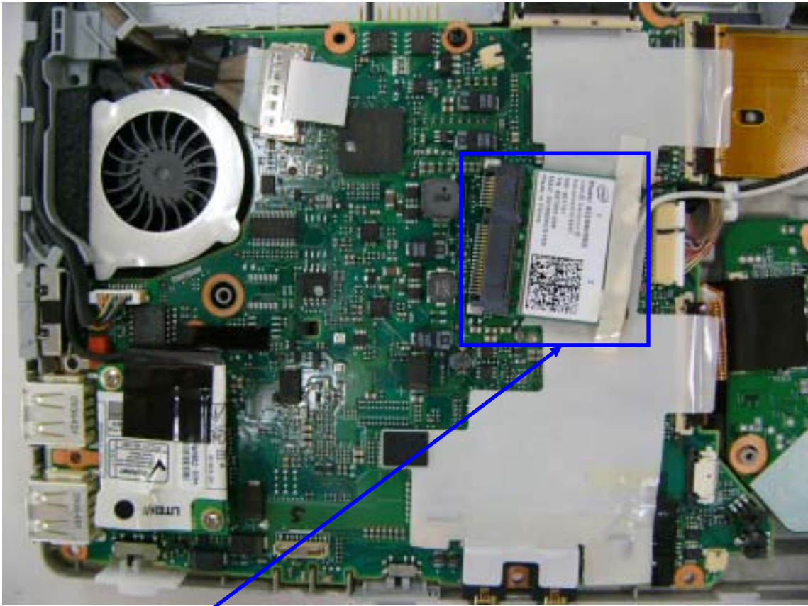
WLAN Module
