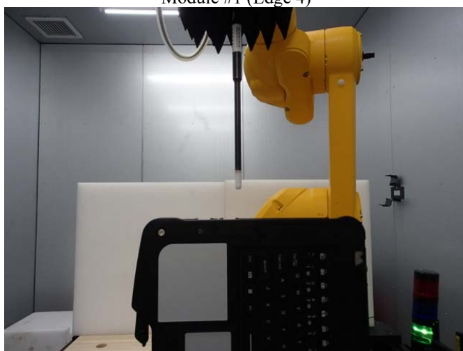
Module #1 (Edge 4)
