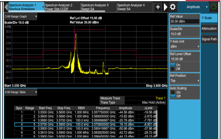
1RB#0 (3575MHz)
