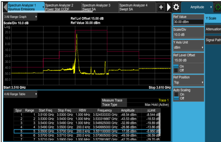
1RB#0 (3560MHz)
