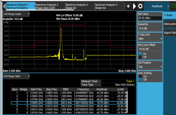
1RB#0 (3590MHz)
