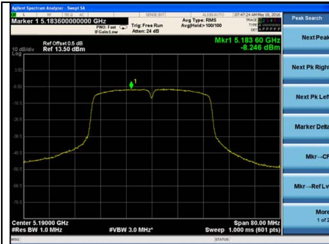
5150-5250MHz PSD - Low CH 5190
