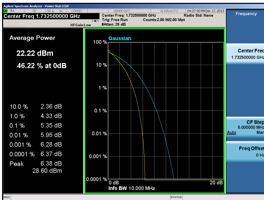
Plot 9-23. PAR Plot (10.0MHz QPSK – RB Size 50)
