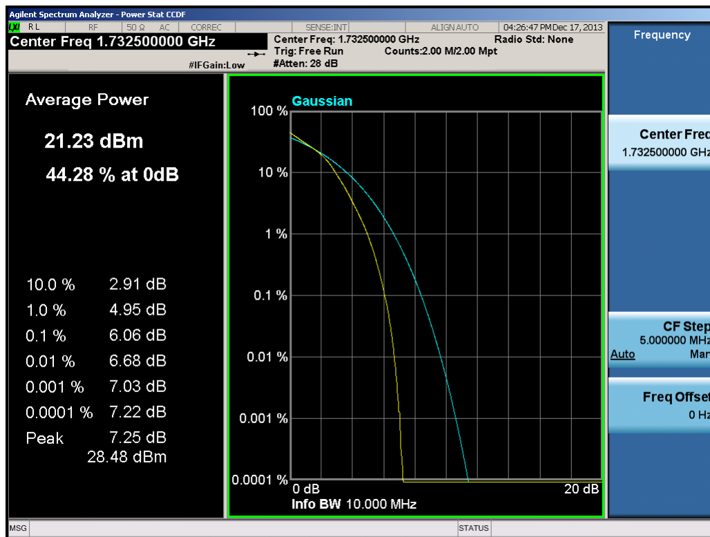
Plot 9-24. PAR Plot (10.0MHz 16-QAM – RB Size 50)
