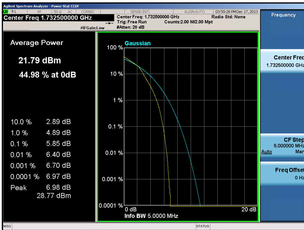
Plot 9-12. PAR Plot (5.0MHz 16-QAM - RB Size 25)
