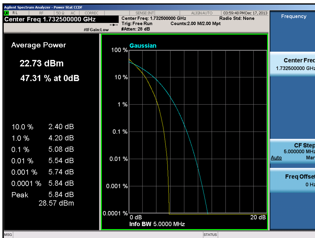
Plot 9-11. PAR Plot (5.0MHz QPSK – RB Size 25)
