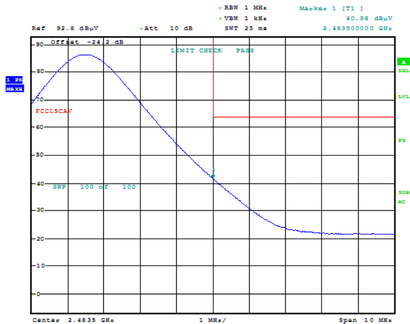
ACJFZN1A BT Upper Band Edge Plot
