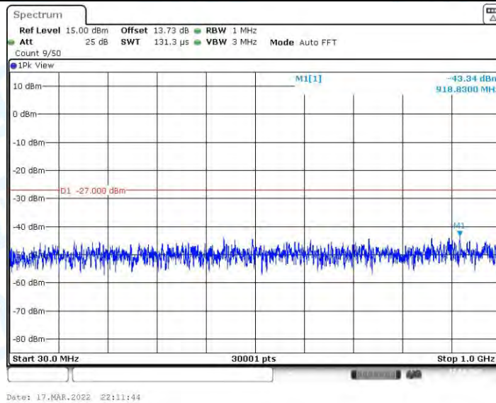
11AX80MIMO_Ant1_5610_30~1000
