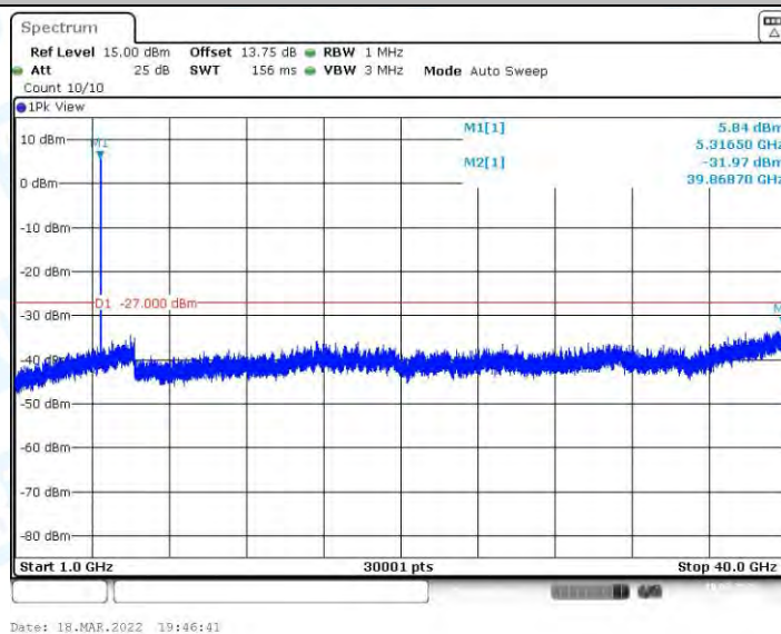
11AX20MIMO_Ant2_5320_1000~40000
