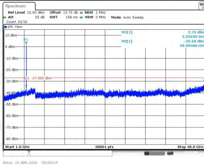
11AX40MIMO_Ant2_5310_1000~40000
