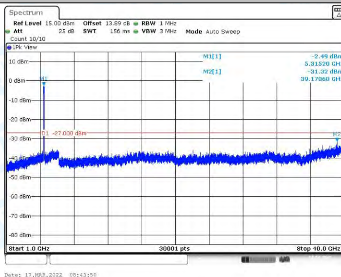
11AX80MIMO_Ant2_5290_1000~40000
