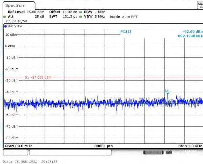
11AX20MIMO_Ant2_5580_30~1000
