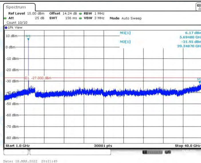
11AX20MIMO_Ant2_5700_1000~40000
