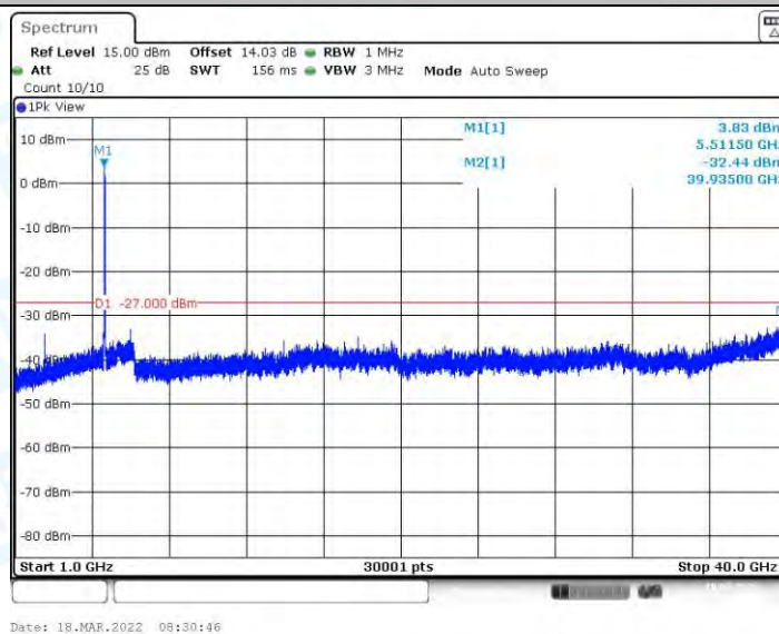
11AX40MIMO_Ant1_5510_1000~40000
