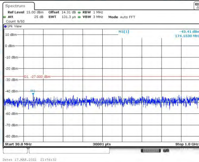
11AX80MIMO_Ant2_5530_30~1000
