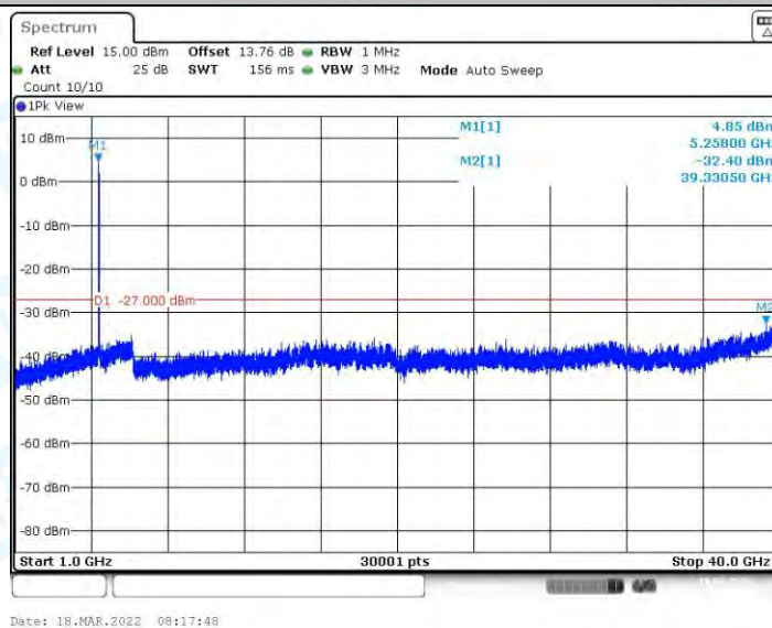
11AX40MIMO_Ant2_5270_1000~40000
