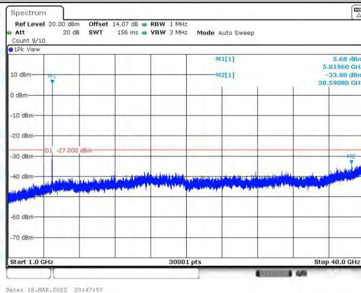
11AX20MIMO_Ant2_5825_1000~40000
