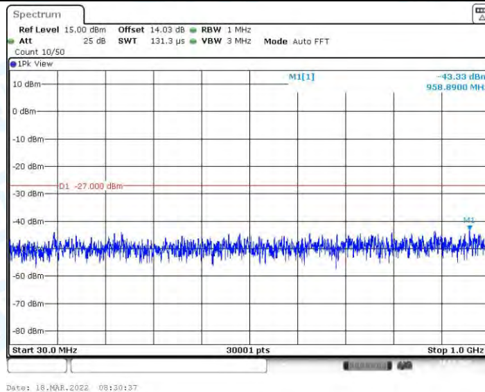
11AX40MIMO_Ant1_5510_30~1000
