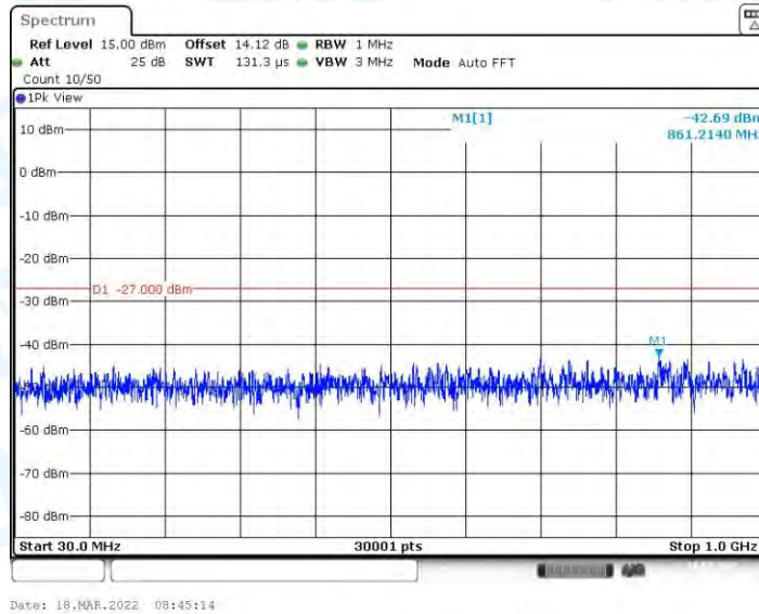
11AX40MIMO_Ant1_5670_30~1000
