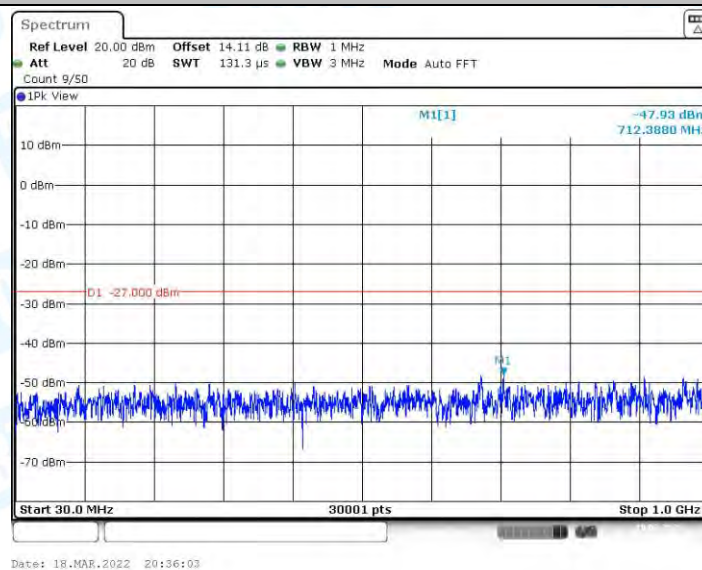
11AX20MIMO_Ant2_5745_30~1000
