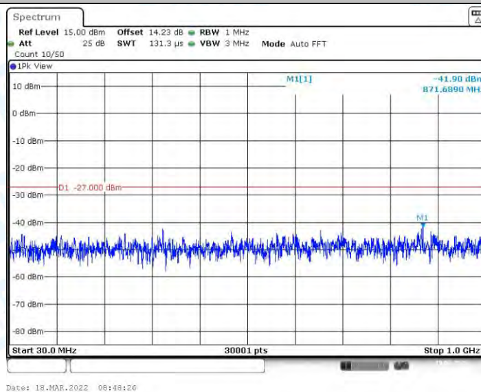
11AX40MIMO_Ant2_5670_30~1000
