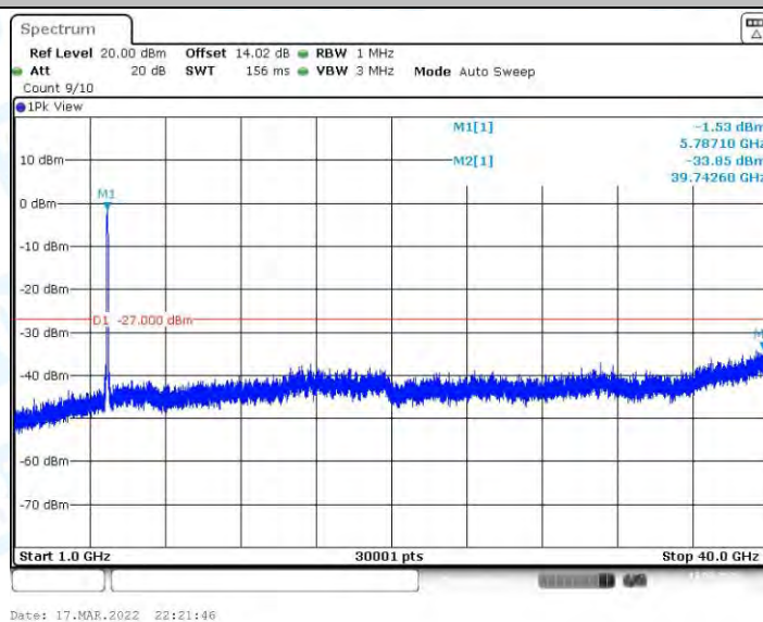
11AX80MIMO_Ant1_5775_1000~40000
