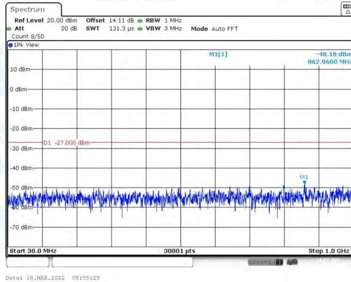
11AX40MIMO_Ant2_5755_30~1000
