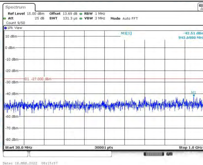
11AX40MIMO_Ant1_5270_30~1000
