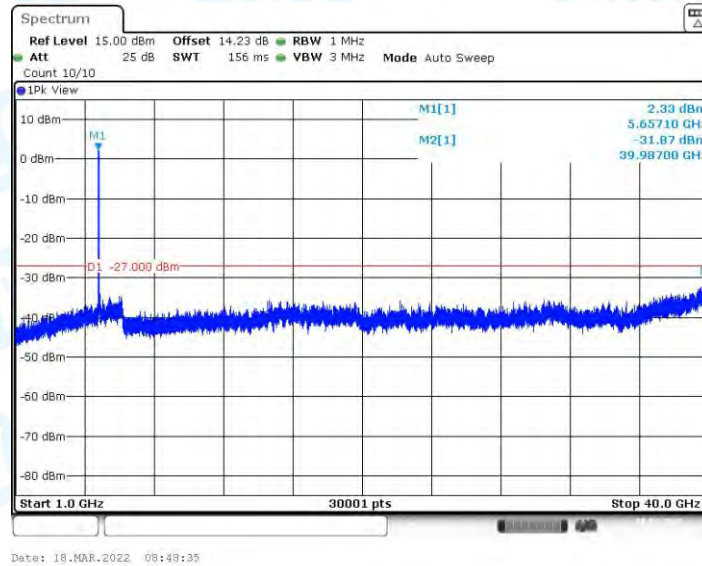
11AX40MIMO_Ant2_5670_1000~40000
