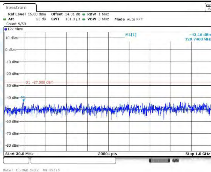
11AX40MIMO_Ant1_5550_30~1000
