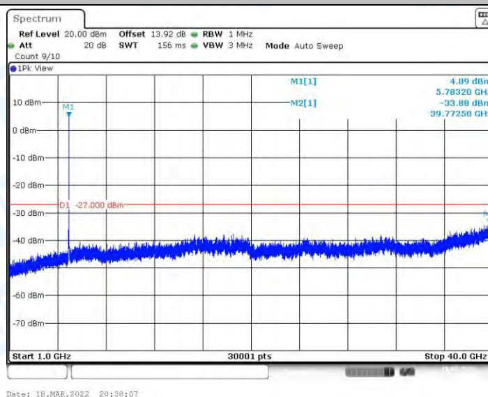
11AX20MIMO_Ant1_5785_1000~40000
