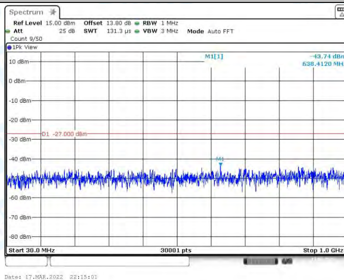
11AX80MIMO_Ant2_5610_30~1000
