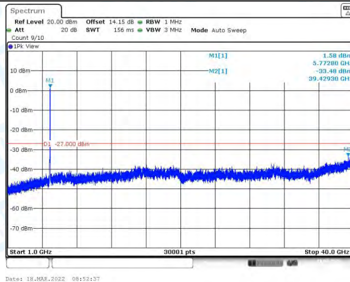
11AX40MIMO_Ant1_5755_1000~40000
