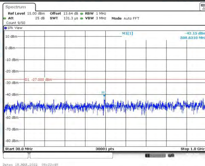
11AX40MIMO_Ant1_5310_30~1000
