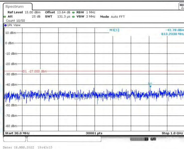
11AX20MIMO_Ant1_5320_30~1000
