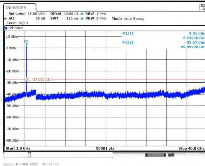
11AX40MIMO_Ant1_5230_1000~40000
