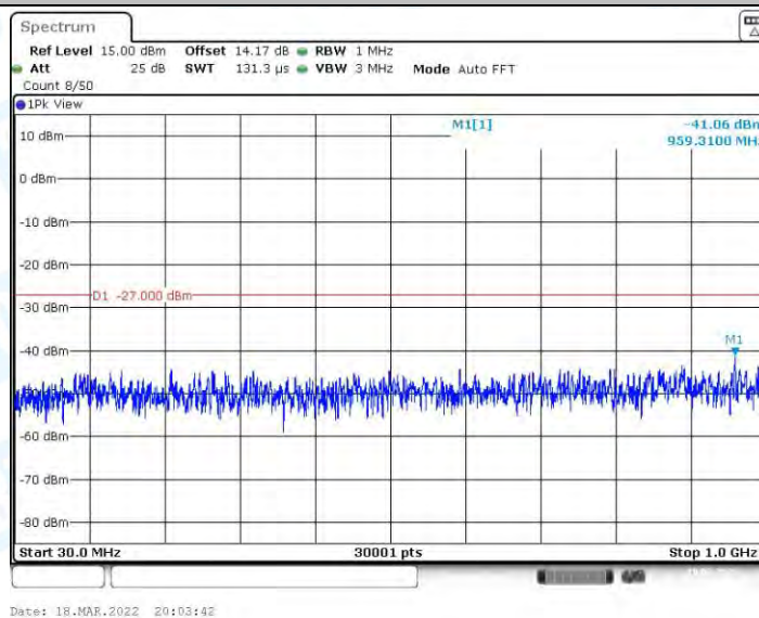
11AX20MIMO_Ant2_5500_30~1000
