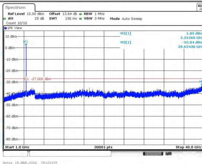
11AX40MIMO_Ant1_5310_1000~40000
