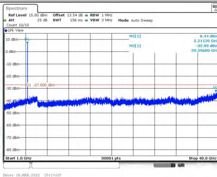
11AX20MIMO_Ant1_5220_1000~40000
