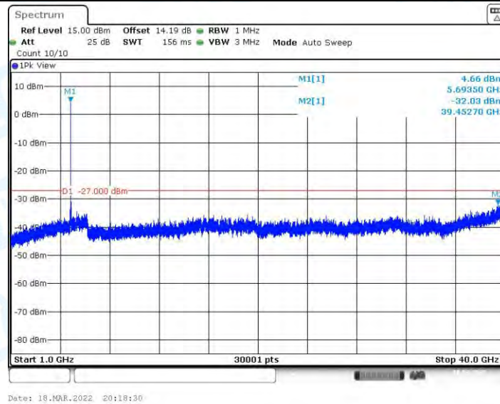
11AX20MIMO_Ant1_5700_1000~40000
