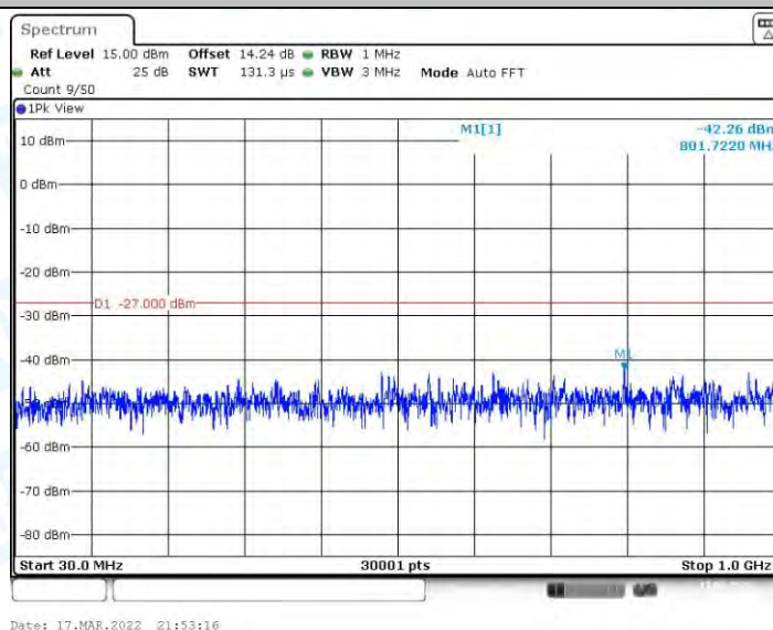
11AX80MIMO_Ant1_5530_30~1000
