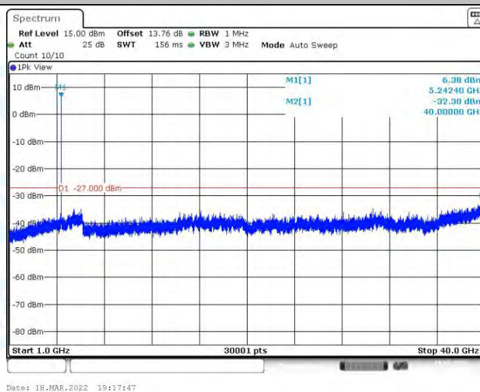
11AX20MIMO_Ant2_5240_1000~40000
