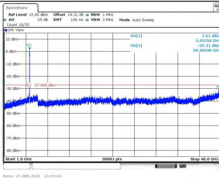
11AX80MIMO_Ant2_5530_1000~40000
