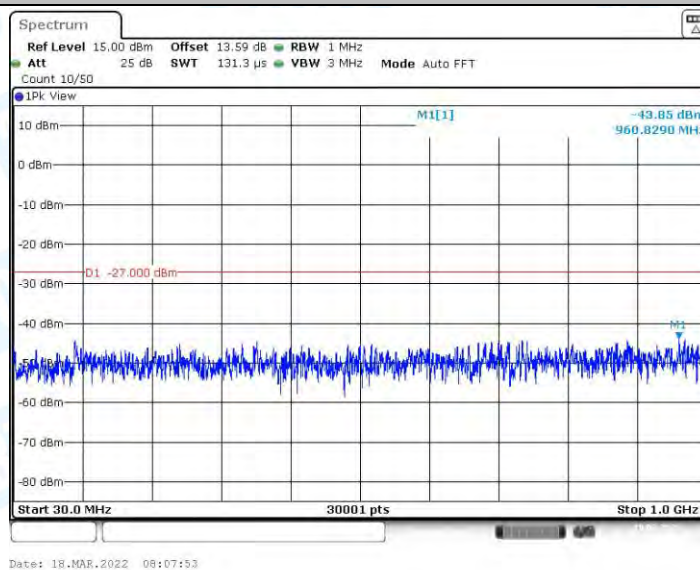
11AX40MIMO_Ant2_5190_30~1000
