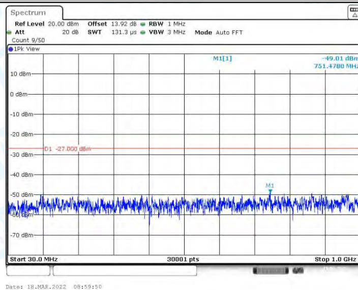
11AX40MIMO_Ant1_5795_30~1000
