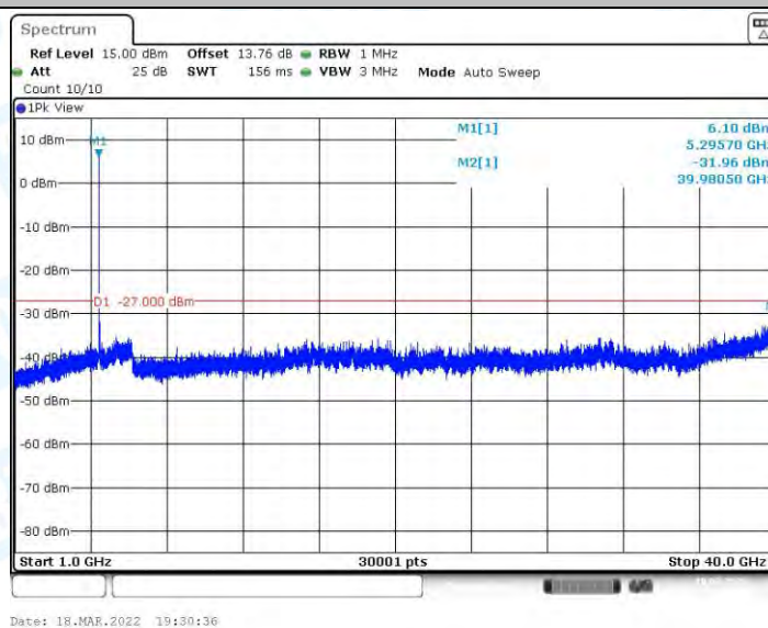
11AX20MIMO_Ant1_5300_1000~40000
