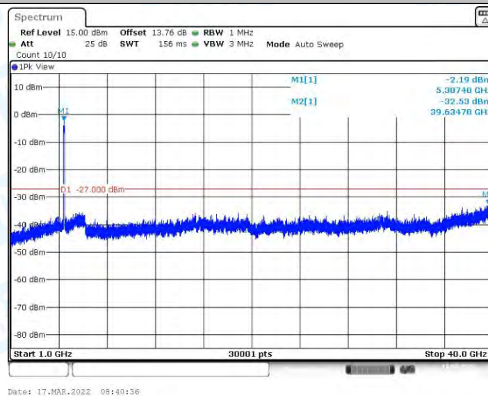
11AX80MIMO_Ant1_5290_1000~40000
