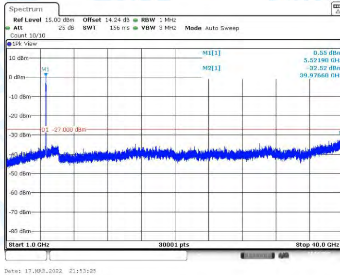
11AX80MIMO_Ant1_5530_1000~40000
