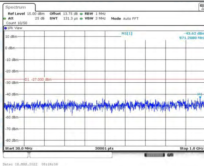
11AX40MIMO_Ant2_5310_30~1000
