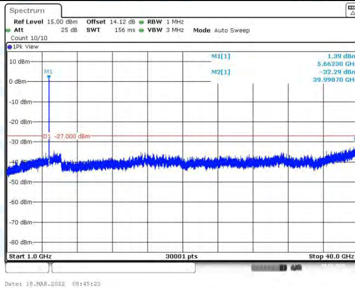
11AX40MIMO_Ant1_5670_1000~40000
