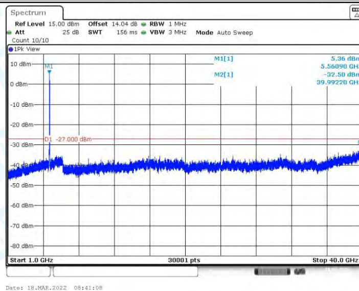
11AX40MIMO_Ant2_5550_1000~40000
