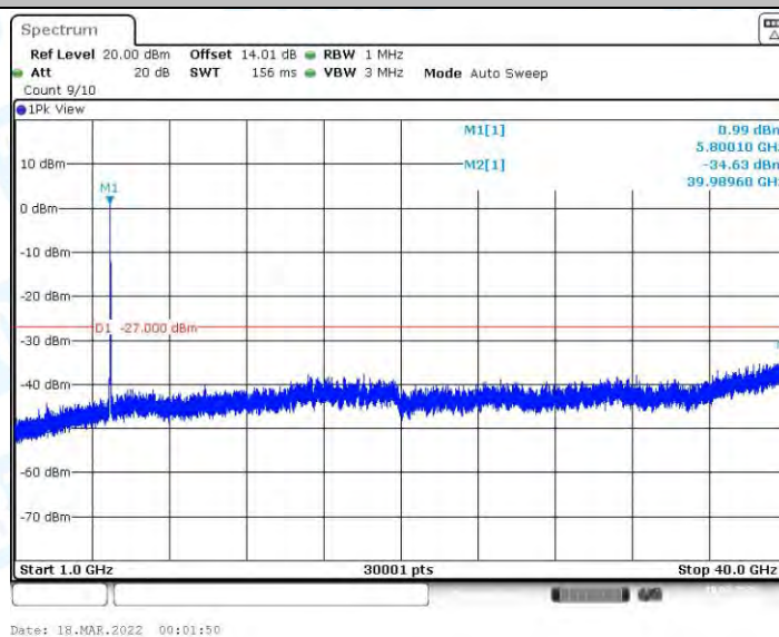
11N40MIMO_Ant2_5795_1000~40000
