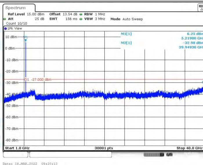
11AC20MIMO_Ant1_5220_1000~40000
