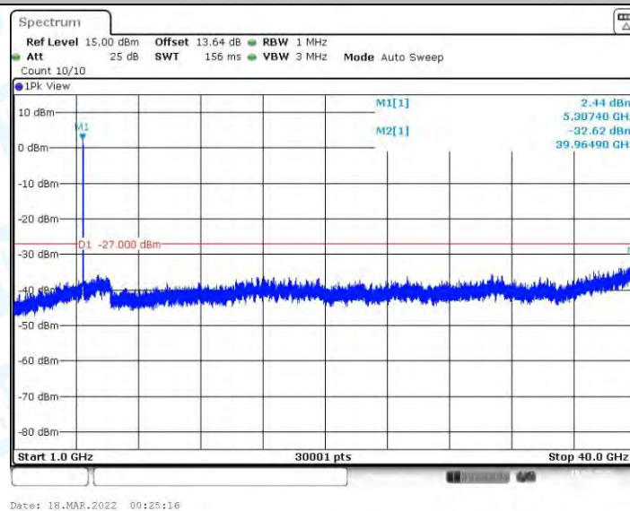
11AC40MIMO_Ant1_5310_1000~40000
