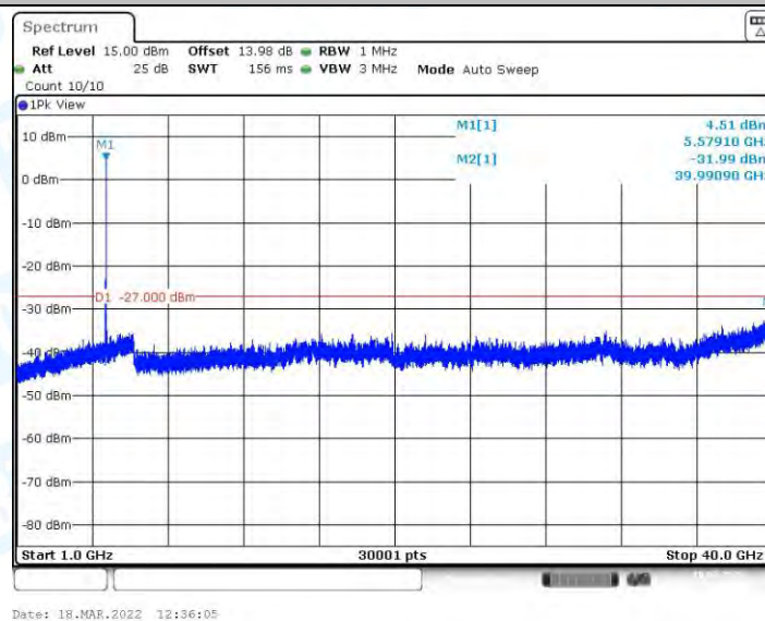
11AC20MIMO_Ant1_5580_1000~40000
