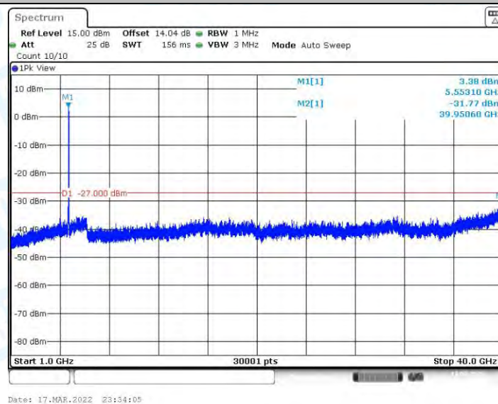
11N40MIMO_Ant2_5550_1000~40000
