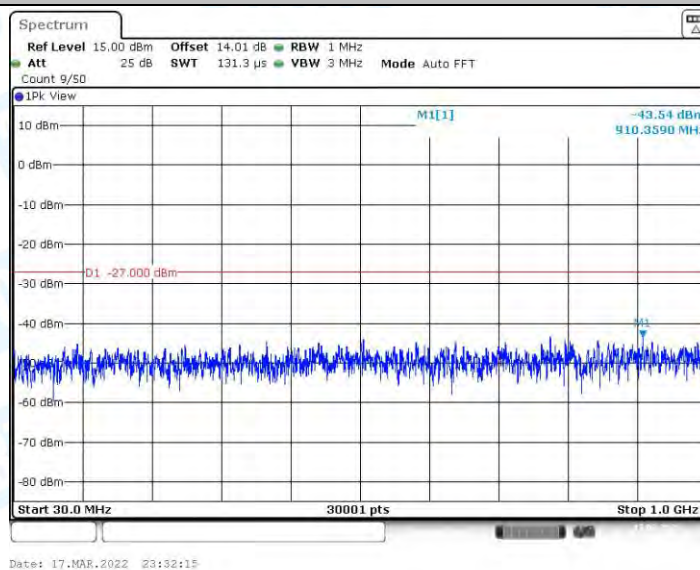
11N40MIMO_Ant1_5550_30~1000
