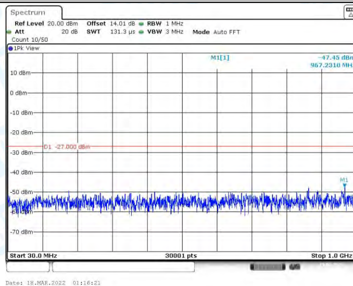
11AC40MIMO_Ant2_5795_30~1000
