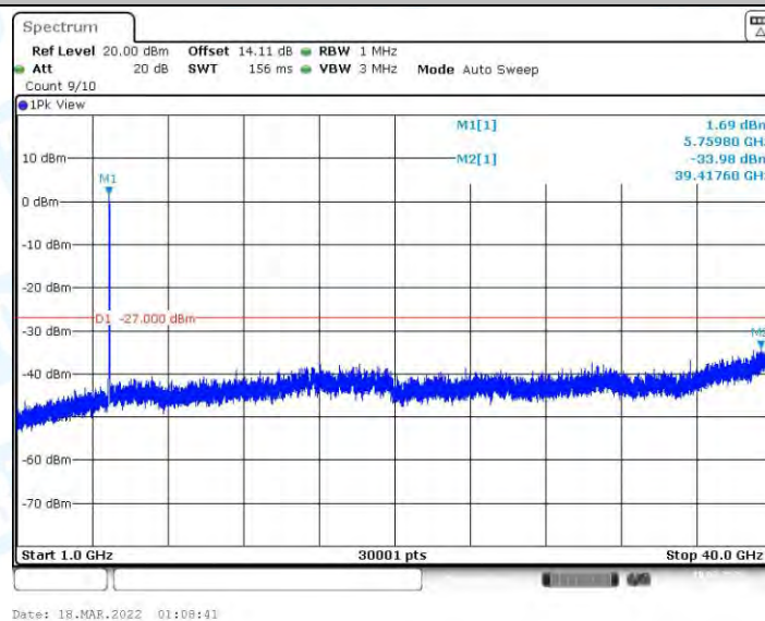
11AC40MIMO_Ant2_5755_1000~40000
