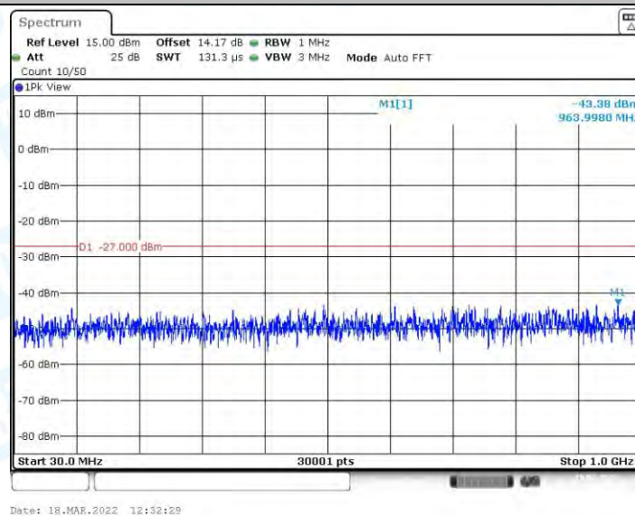
11AC20MIMO_Ant2_5500_30~1000
