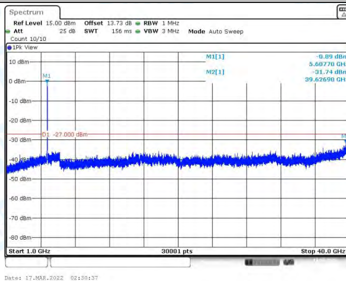
11AC80MIMO_Ant1_5610_1000~40000
