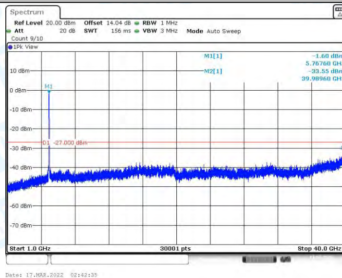
11AC80MIMO_Ant2_5775_1000~40000
