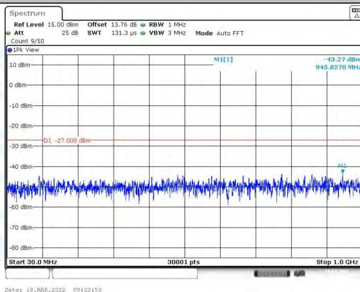
11AC20MIMO_Ant1_5300_30~1000
