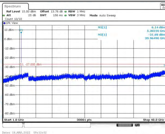
11AC20MIMO_Ant1_5300_1000~40000
