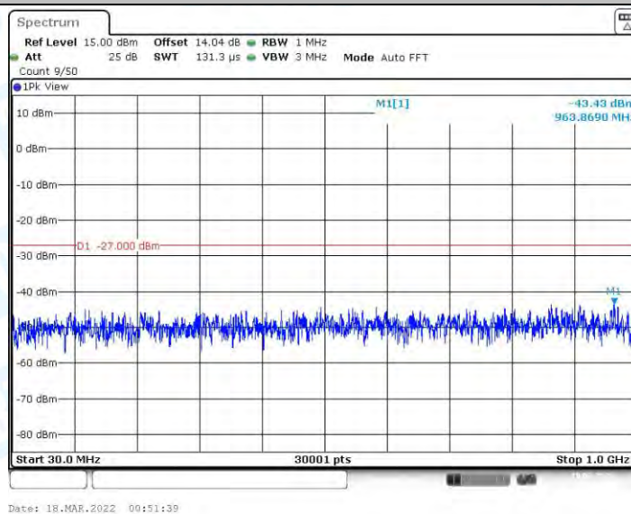
11AC40MIMO_Ant2_5550_30~1000
