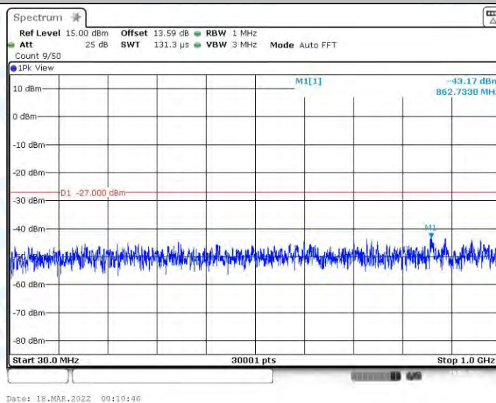
11AC40MIMO_Ant2_5190_30~1000
