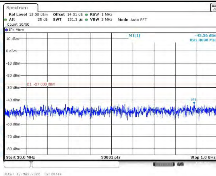
11AC80MIMO_Ant2_5530_30~1000
