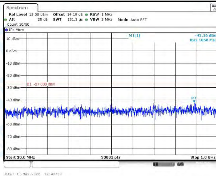
11AC20MIMO_Ant1_5700_30~1000
