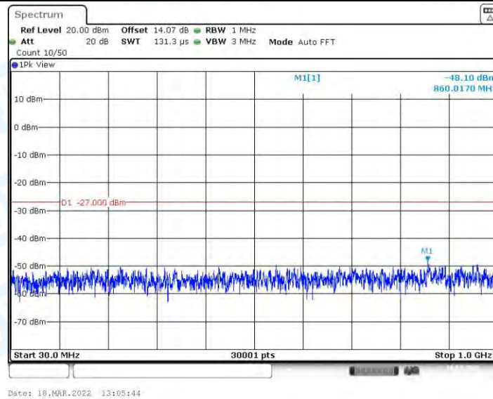
11AC20MIMO_Ant2_5825_30~1000
