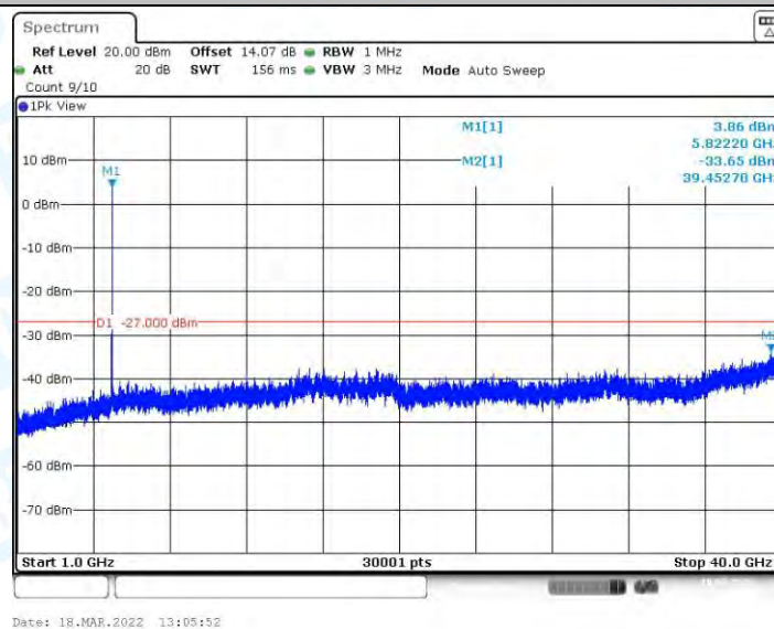
11AC20MIMO_Ant2_5825_1000~40000
