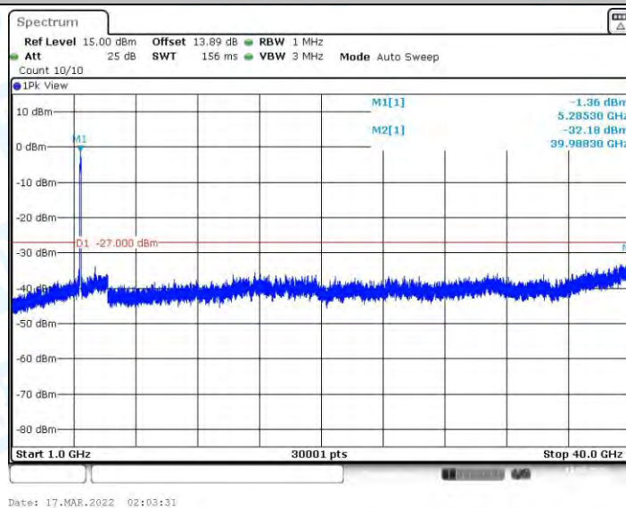
11AC80MIMO_Ant2_5290_1000~40000
