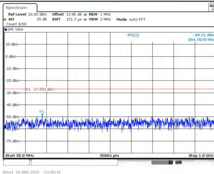
11AC20MIMO_Ant1_5825_30~1000
