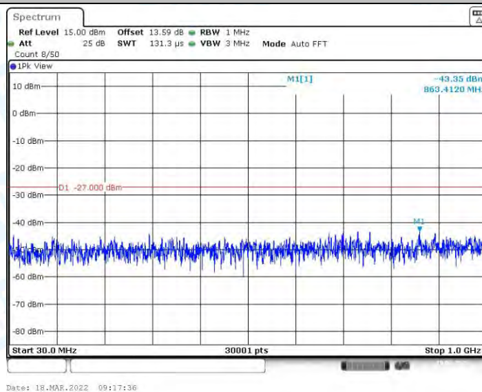
11AC20MIMO_Ant2_5180_30~1000
