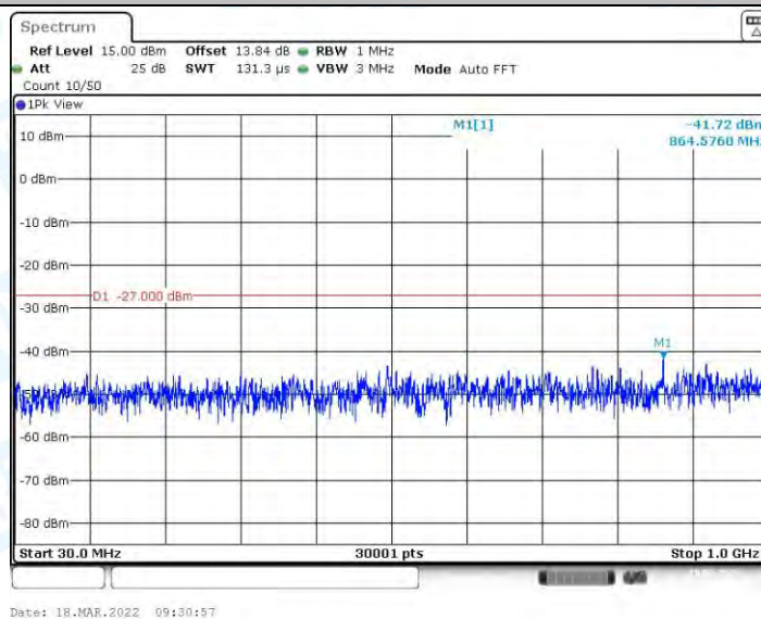
11AC20MIMO_Ant2_5260_30~1000
