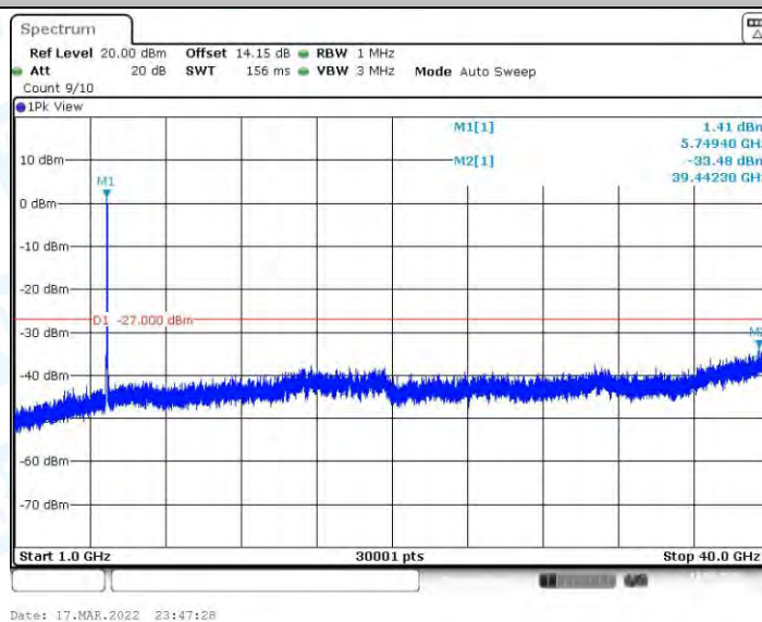
11N40MIMO_Ant1_5755_1000~40000
