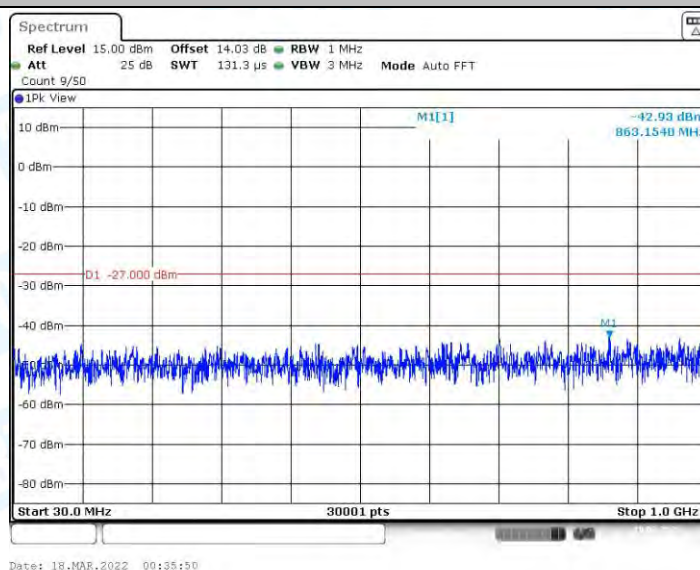
11AC40MIMO_Ant1_5510_30~1000
