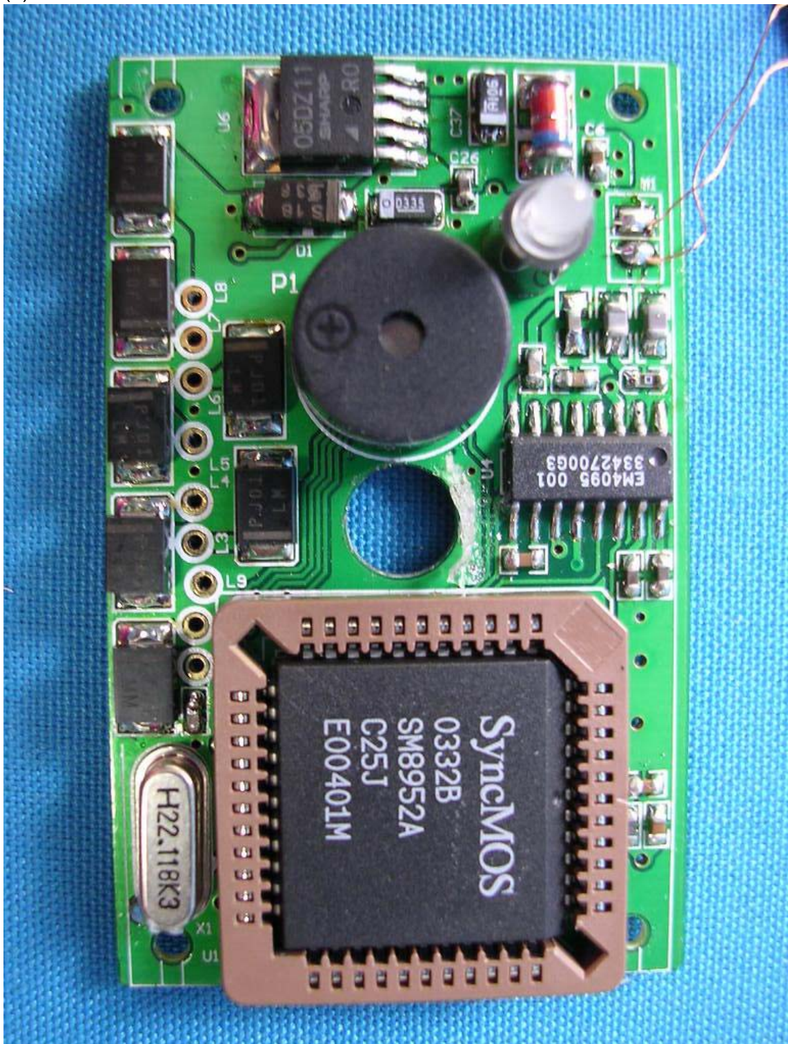
(6) EUT Photo
