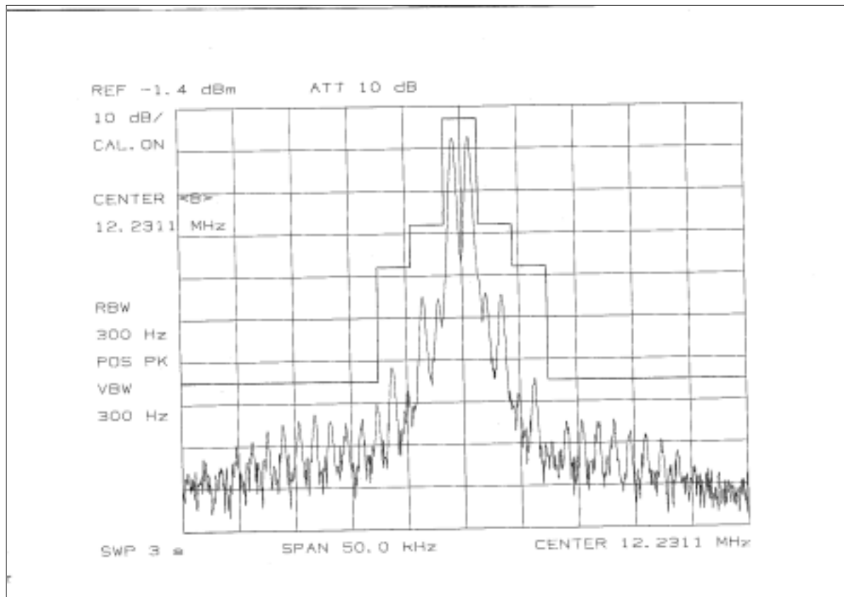
Fig. 3.3.8 - (Fc: 12 MHz, J3E)
