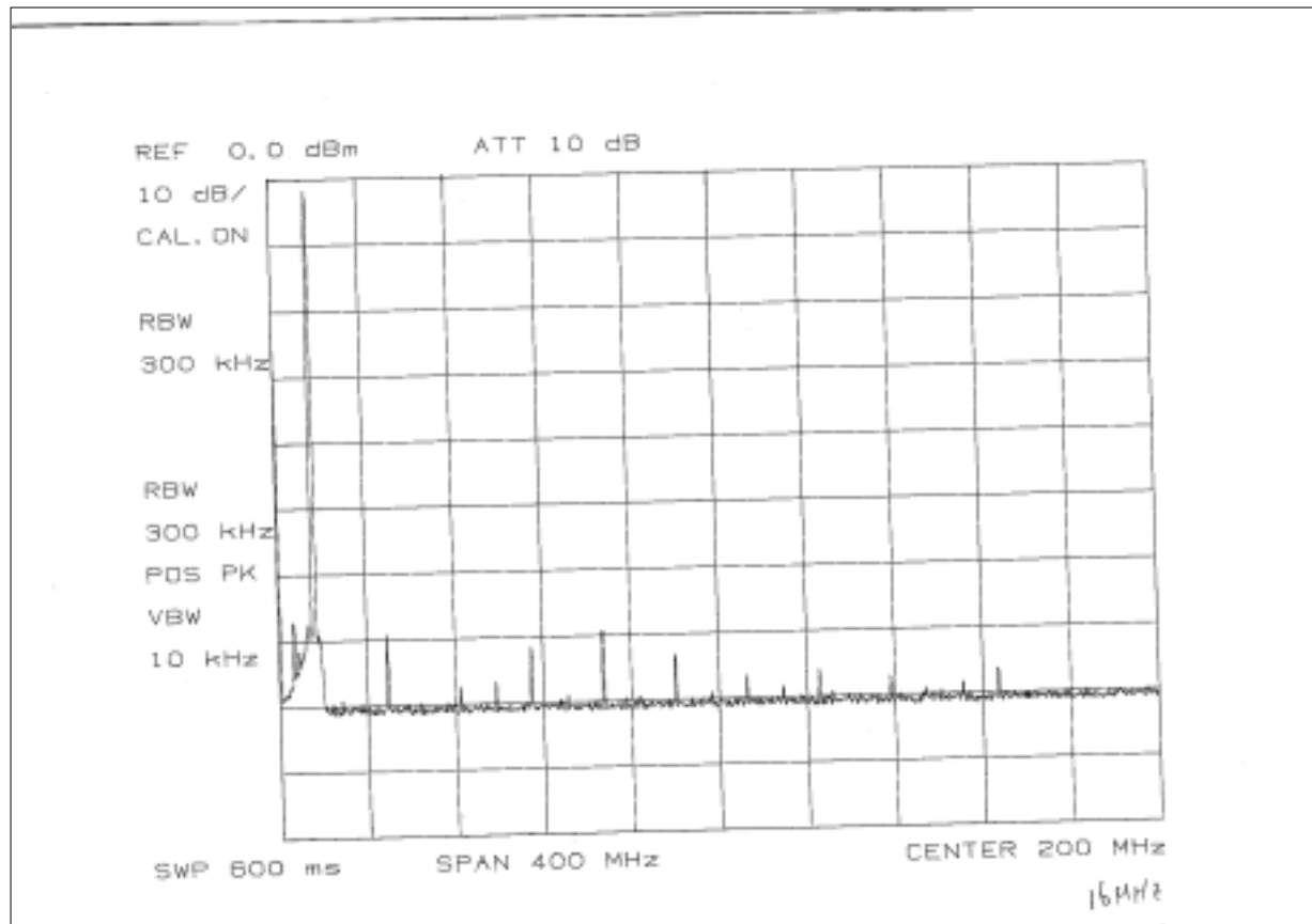
Fig. 3.5.18 - (Fc: 16360 kHz, J3E)
