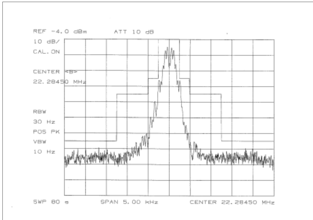
Fig. 3.3.21 - (Fc: 22 MHz, F1B/J2B)
