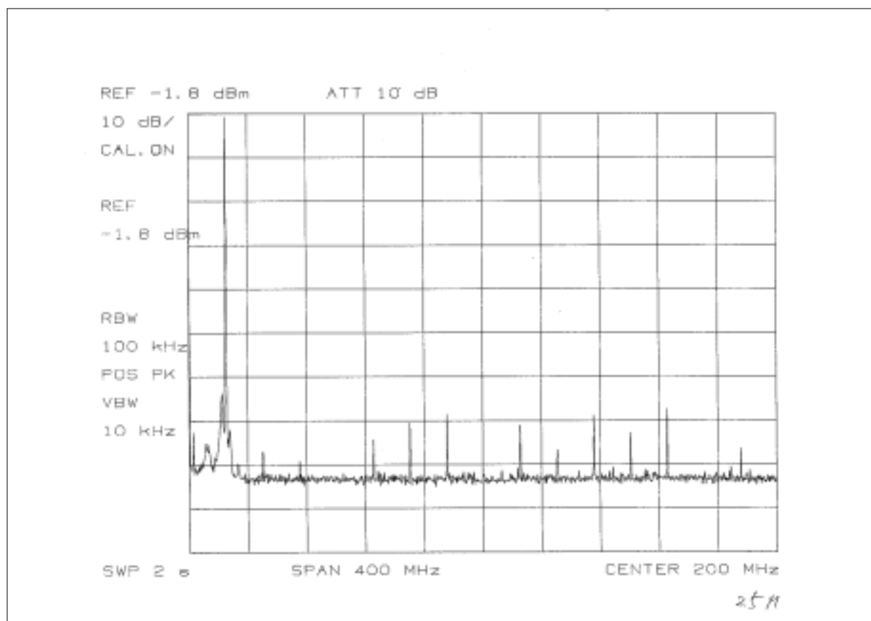
Fig. 3.5.24 - (Fc: 25700 kHz, J3E)
