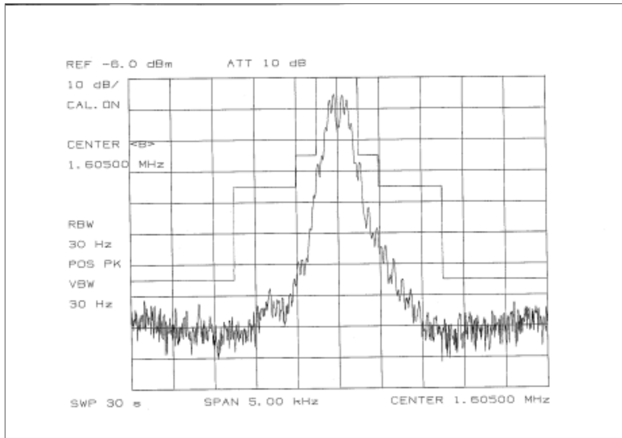
Fig. 3.3.13 - (Fc: 1.6 MHz, F1B/J2B)
