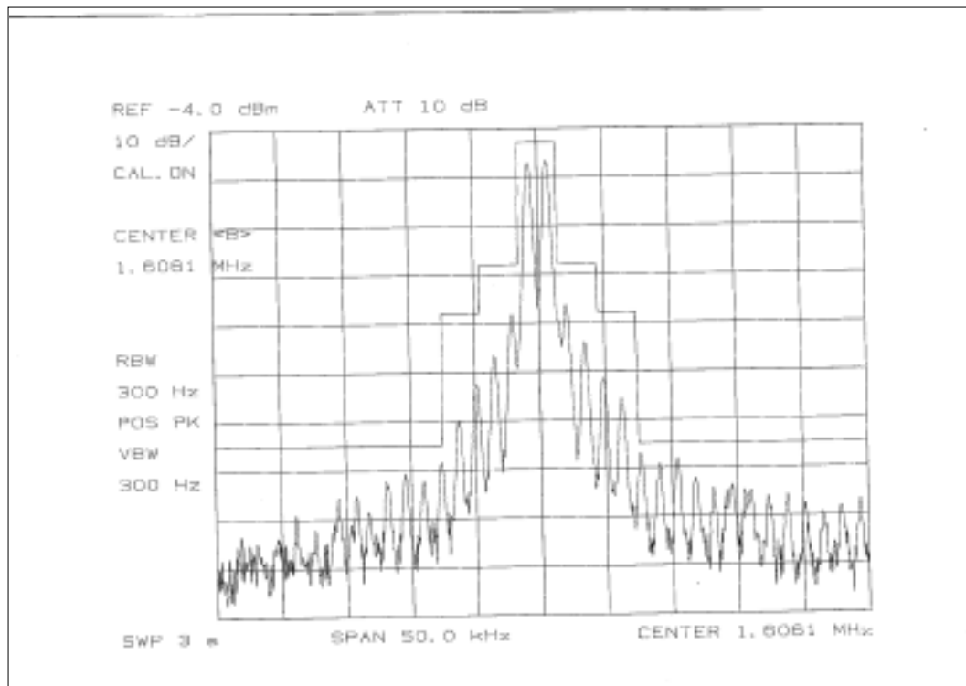
Fig. 3.3.2 - (Fc: 1.6 MHz, J3E)
