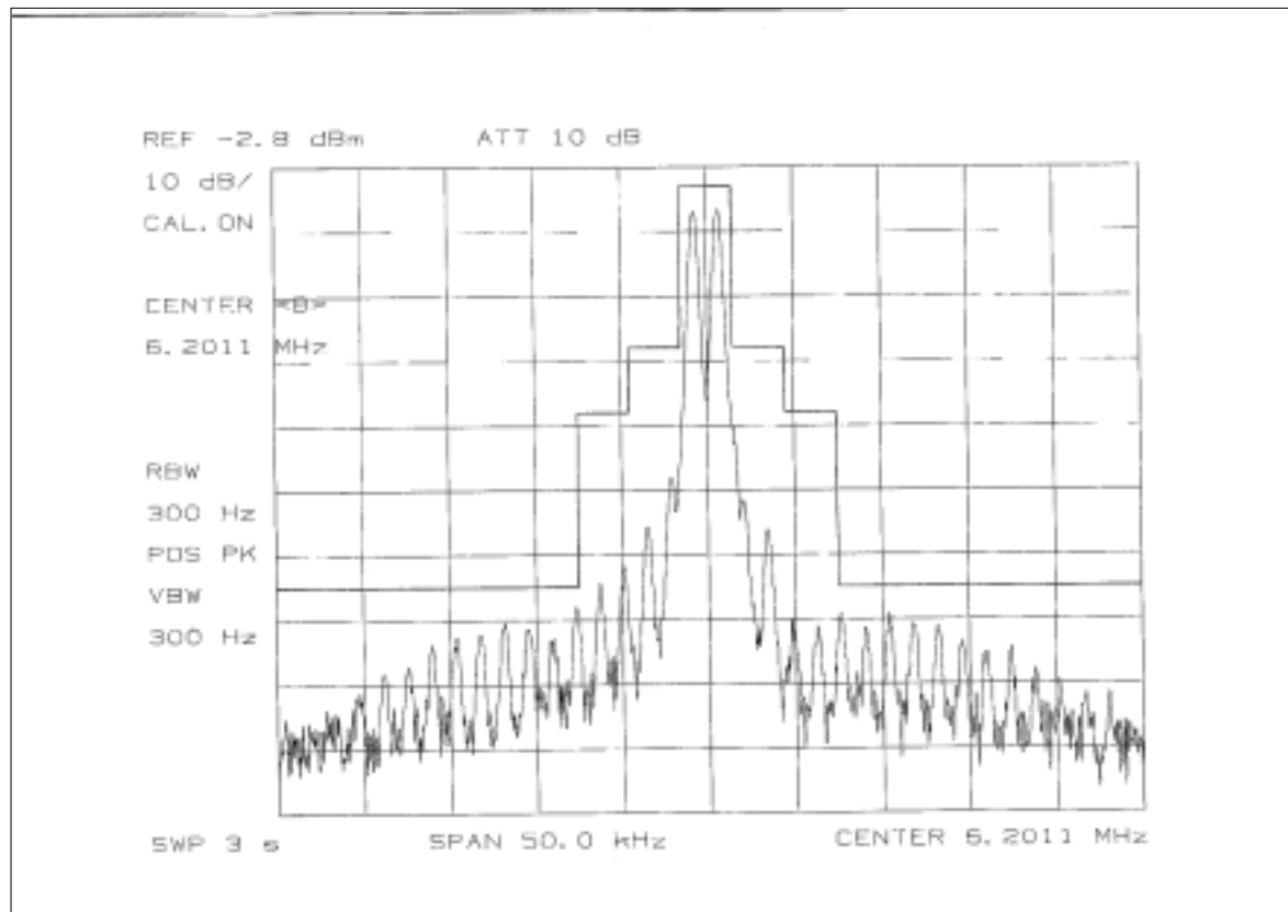
Fig. 3.3.6 - (Fc: 6 MHz, J3E)
