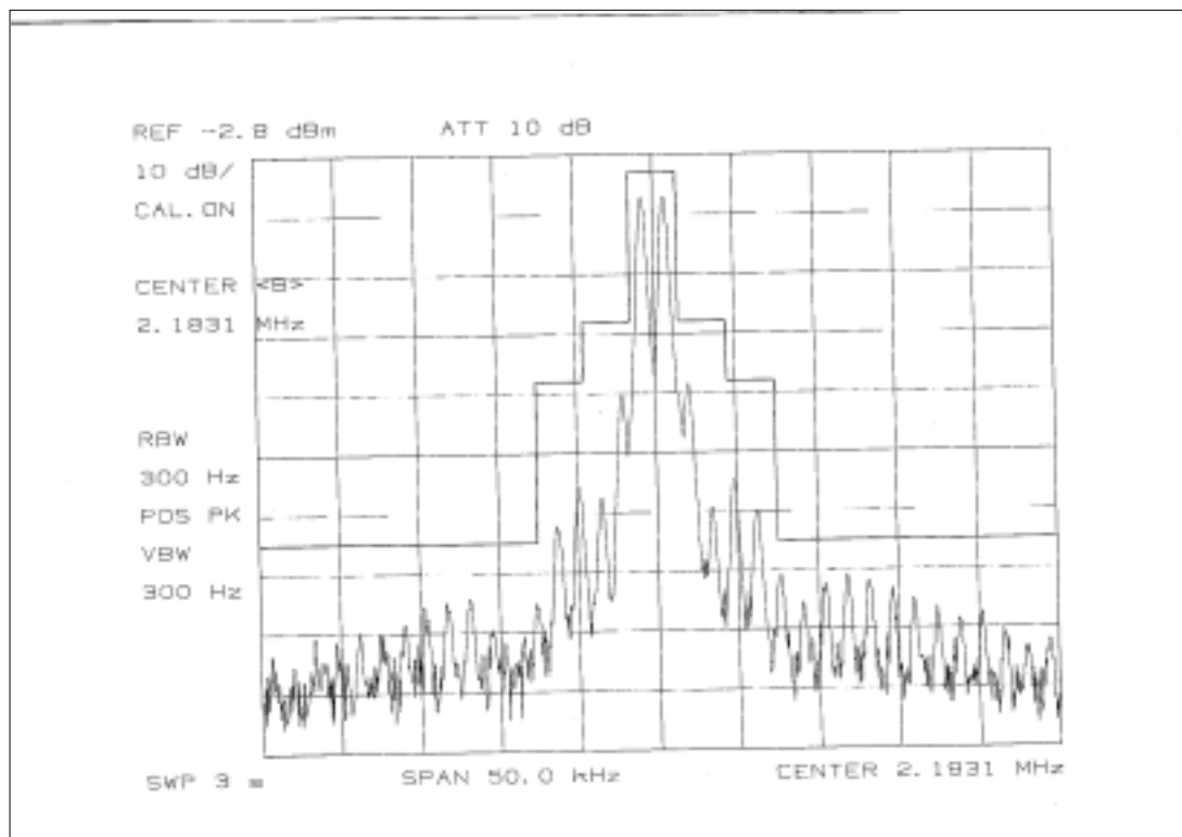
Fig. 3.3.3 - (Fc: 2 MHz, J3E)
