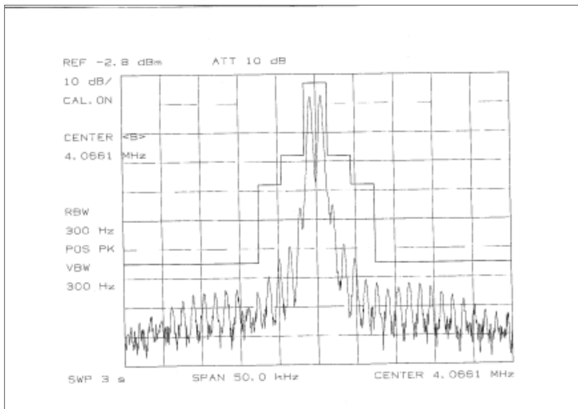
Fig. 3.3.5 - (Fc: 4 MHz, J3E)
