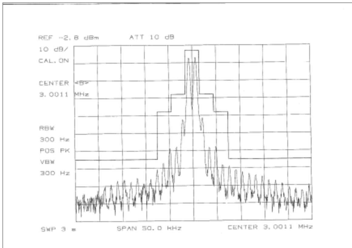
Fig. 3.3.4 - (Fc: 3 MHz, J3E)
