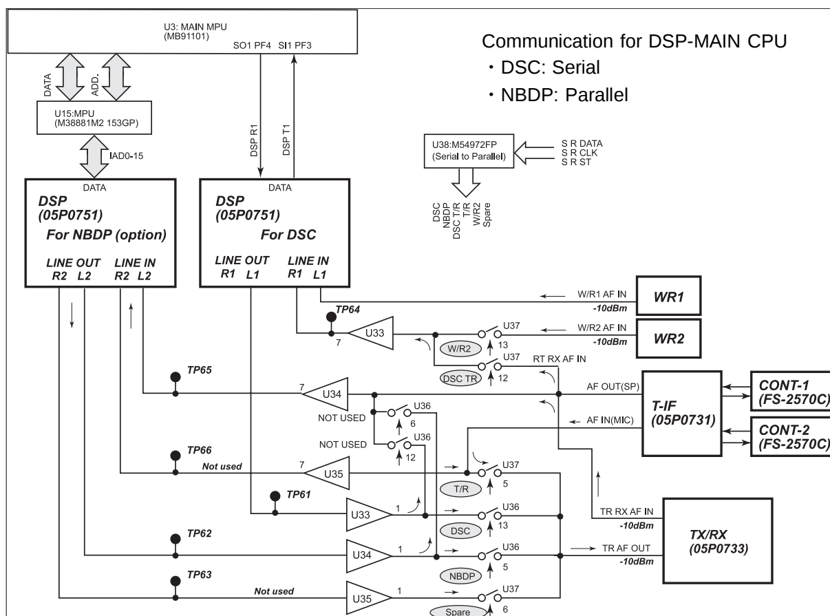
Fig.6.2.3.1-3 DSP input/output circuit
