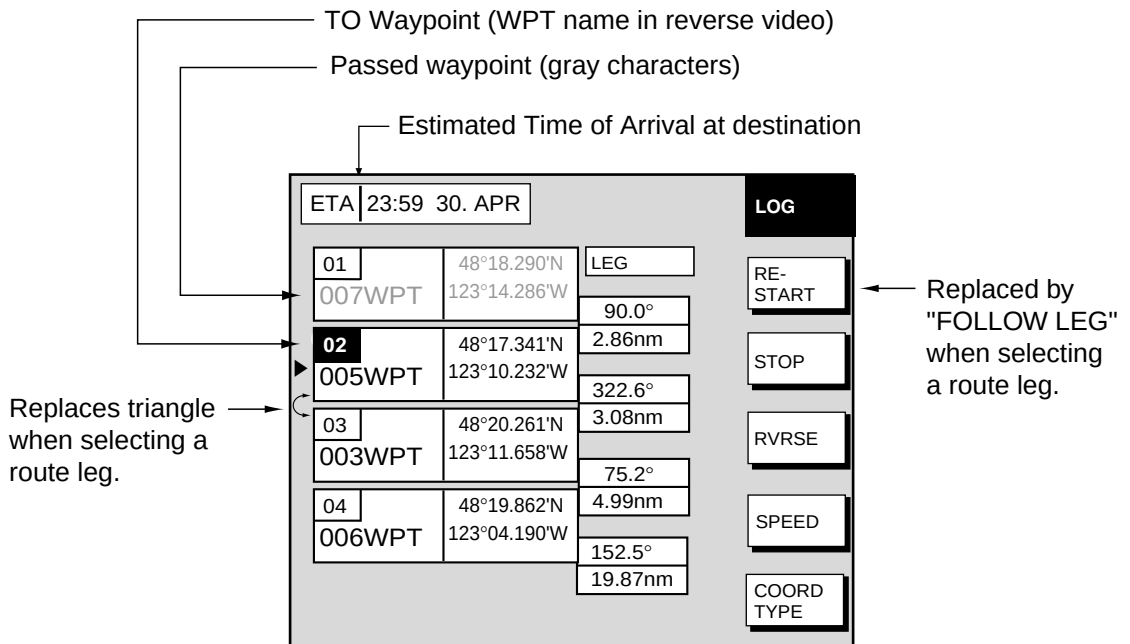
Log display
