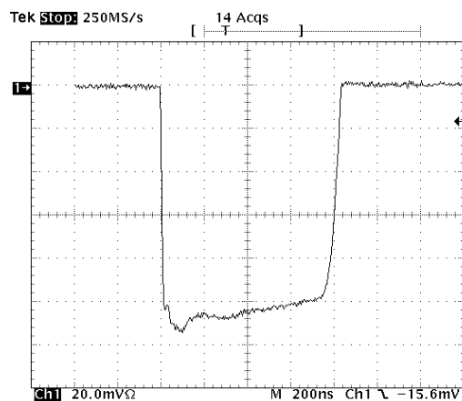
Fig. 3.2.3.4 Long Pulse (48 nm Range) Scale: 20 mV/div. 200 ns/div.
