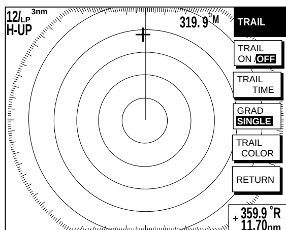
Radar Display
