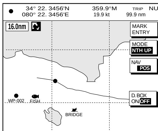
Plotter Display
