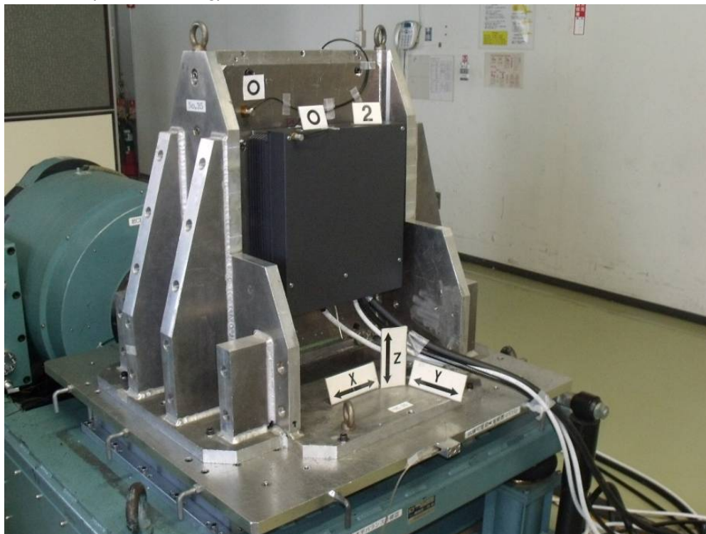
PSU-014 (Wall-mounting)
