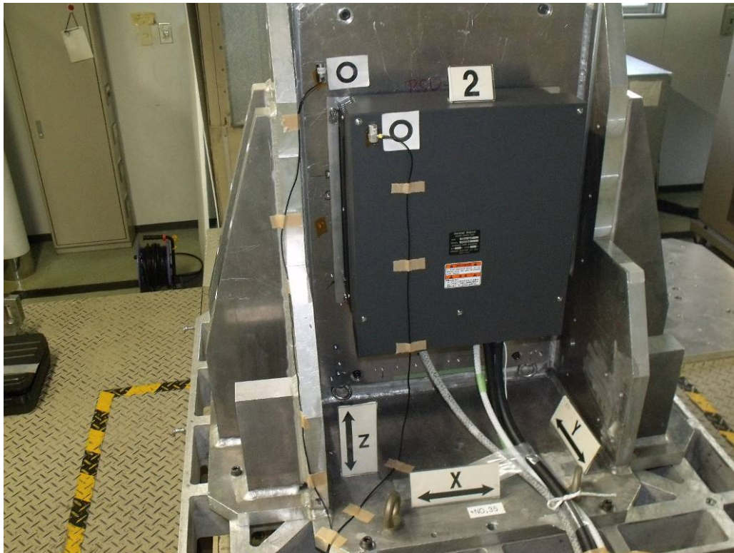
PSU-015 (Wall-mounting),
