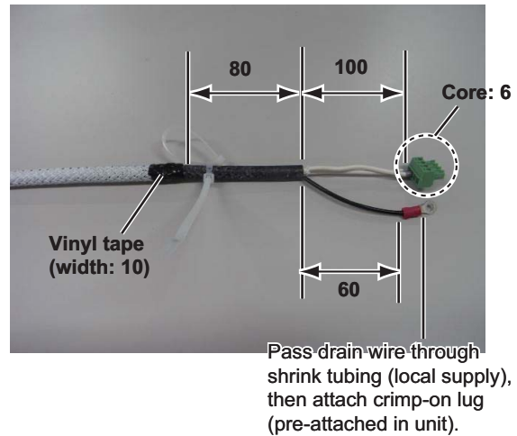
TTYCSLA-1 cable
