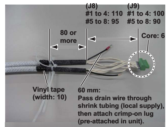
TTYCSLA-1Q cable
