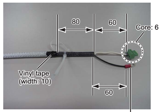
TTYCSLA-1 (MC-3010A)
