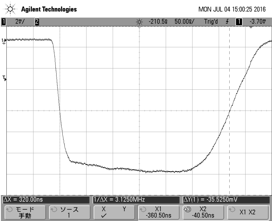
Fig. 7.3 M1 Pulse Envelope
