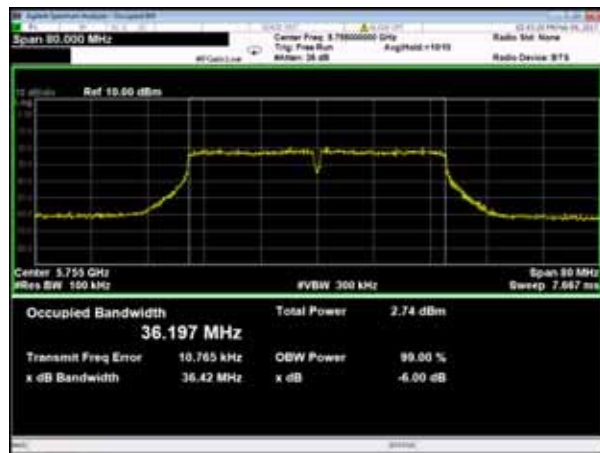
5755MHz
