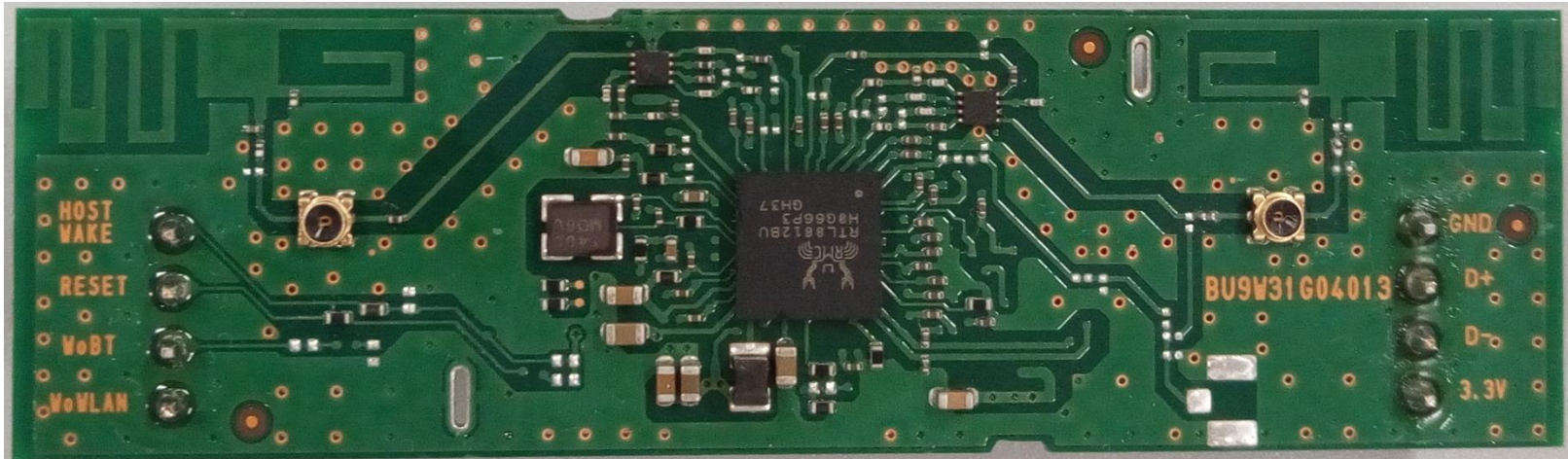
Top Side
