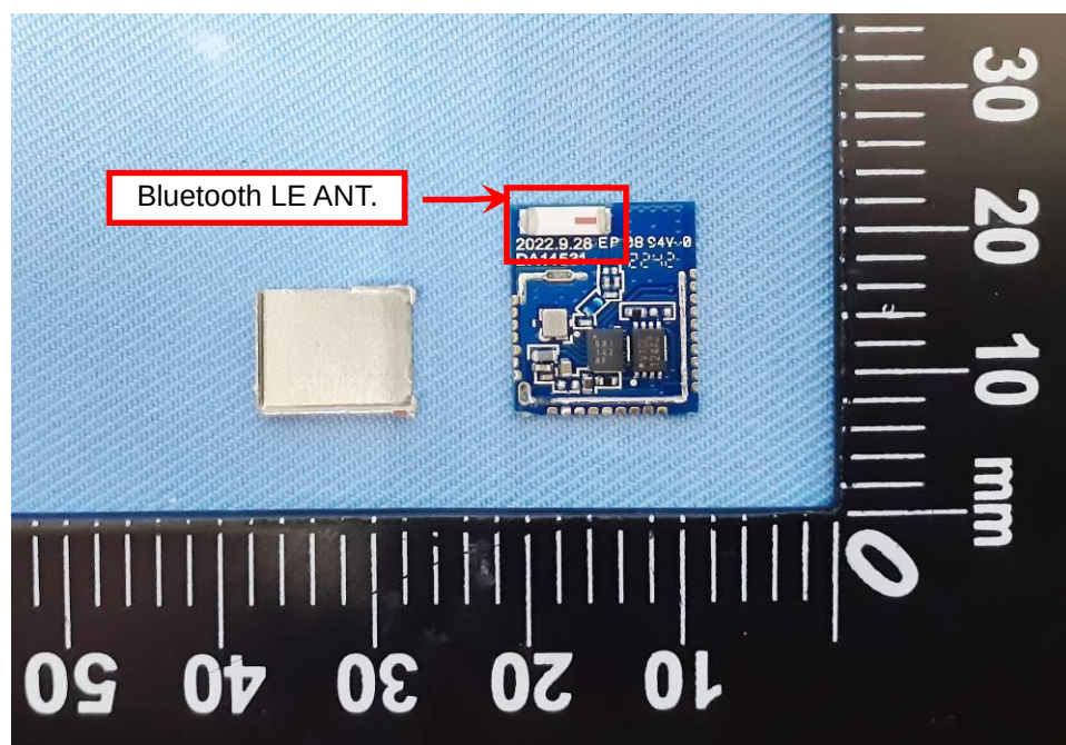
EUT Photo (2)
