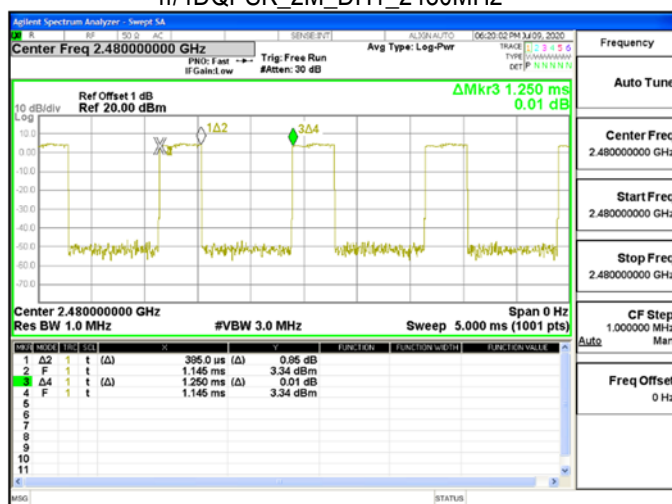
\pi/4 DQPSK_2M_DH1_2480MHz
